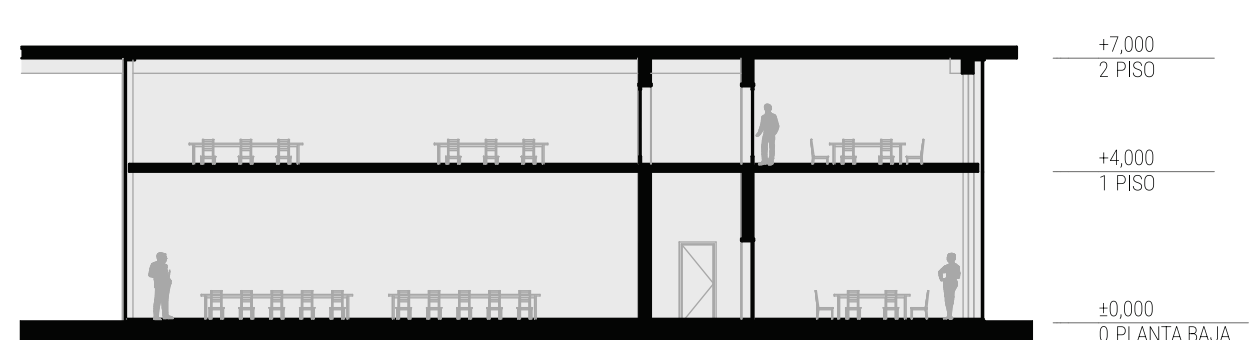
Corte CC - Esc 1:200
