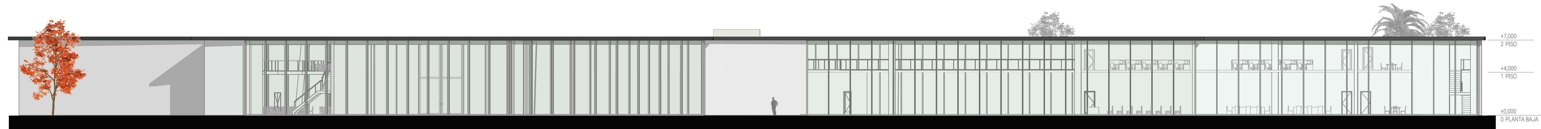
Vista Este - Esc 1:200
