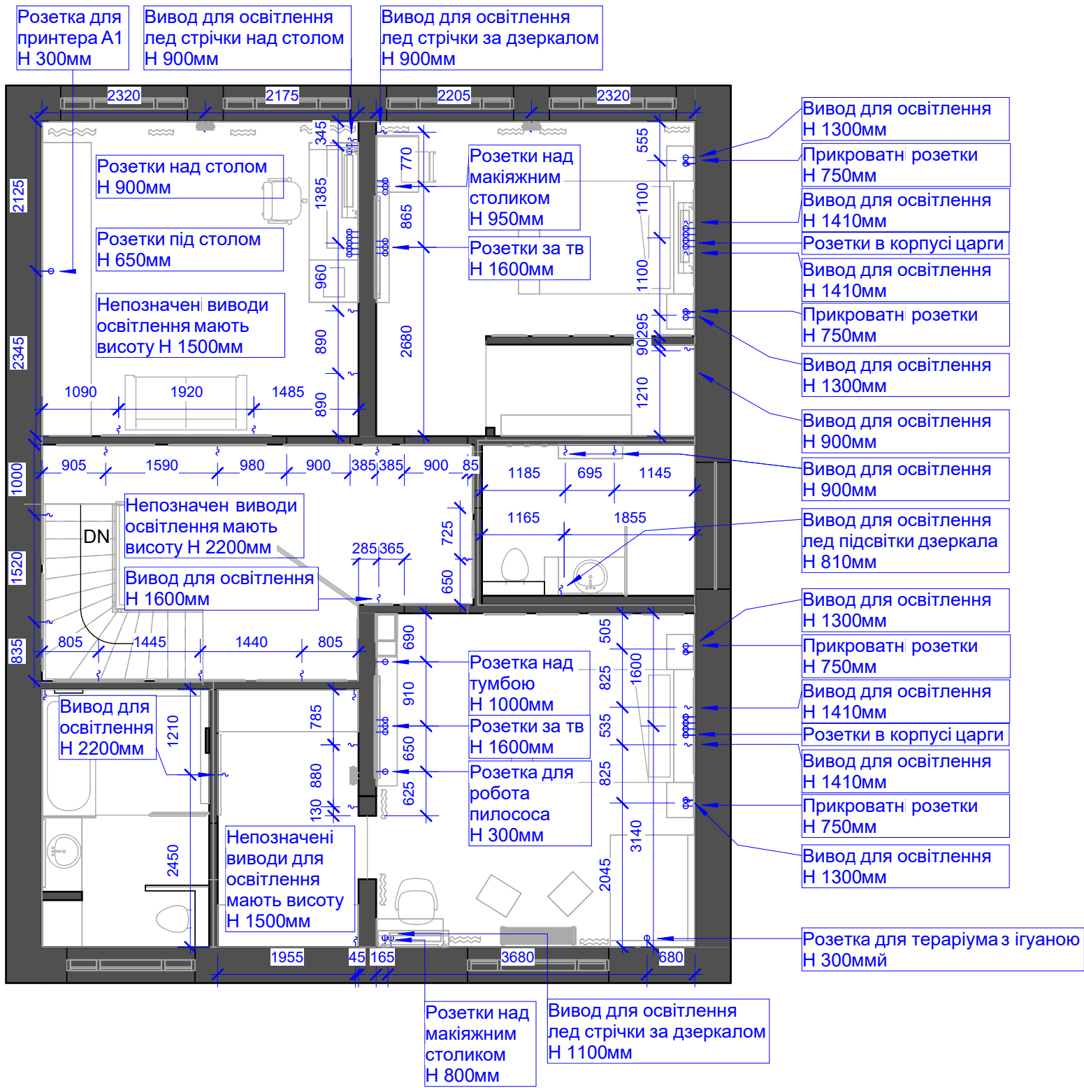
Level 2 Електрика розетки
