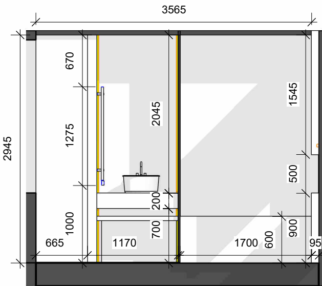
Level 2 Маркування Головна ванна
