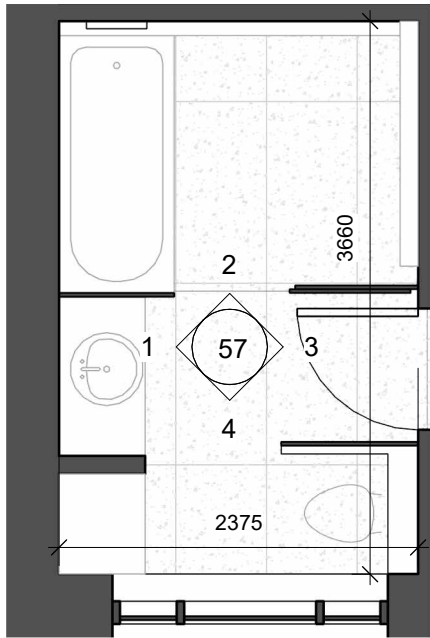
Level 2 Маркування Головна ванна
