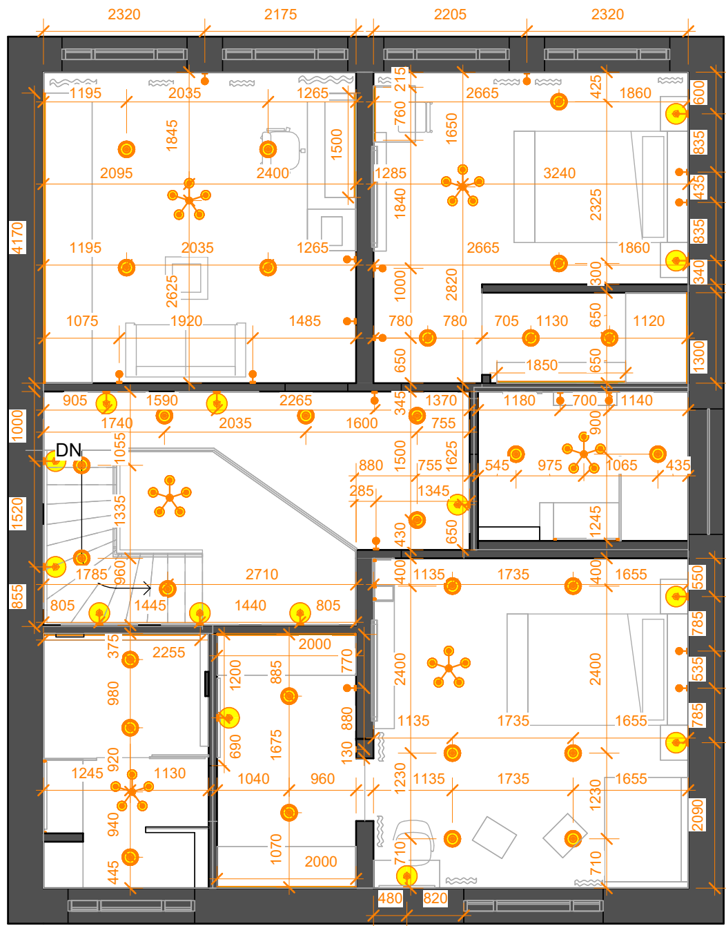
Level 2 План освітлення
