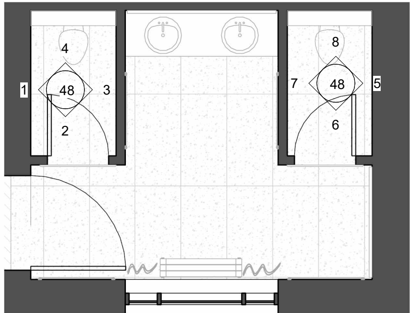
Level 1 Маркування Туалет 1
