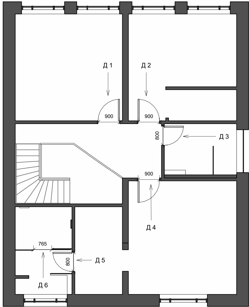
Level 2 План дверей
