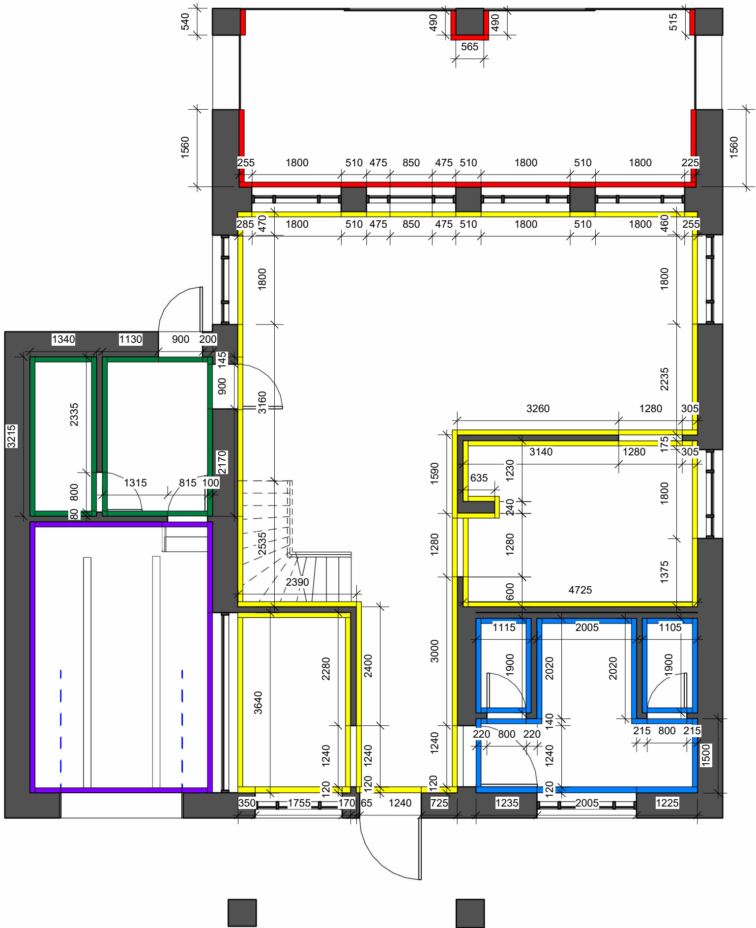
Level 1 План оздоблення стін
