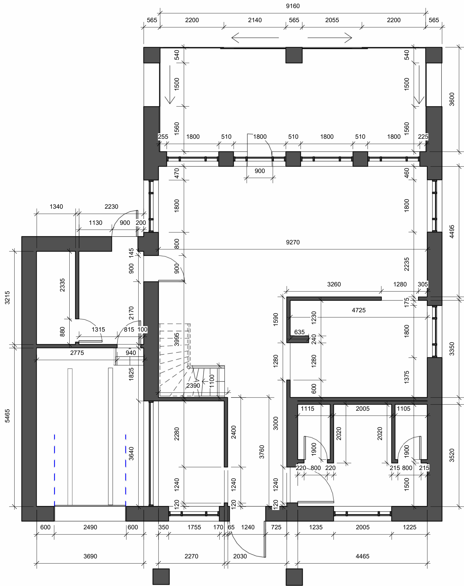
Level 1 Після перепланування
