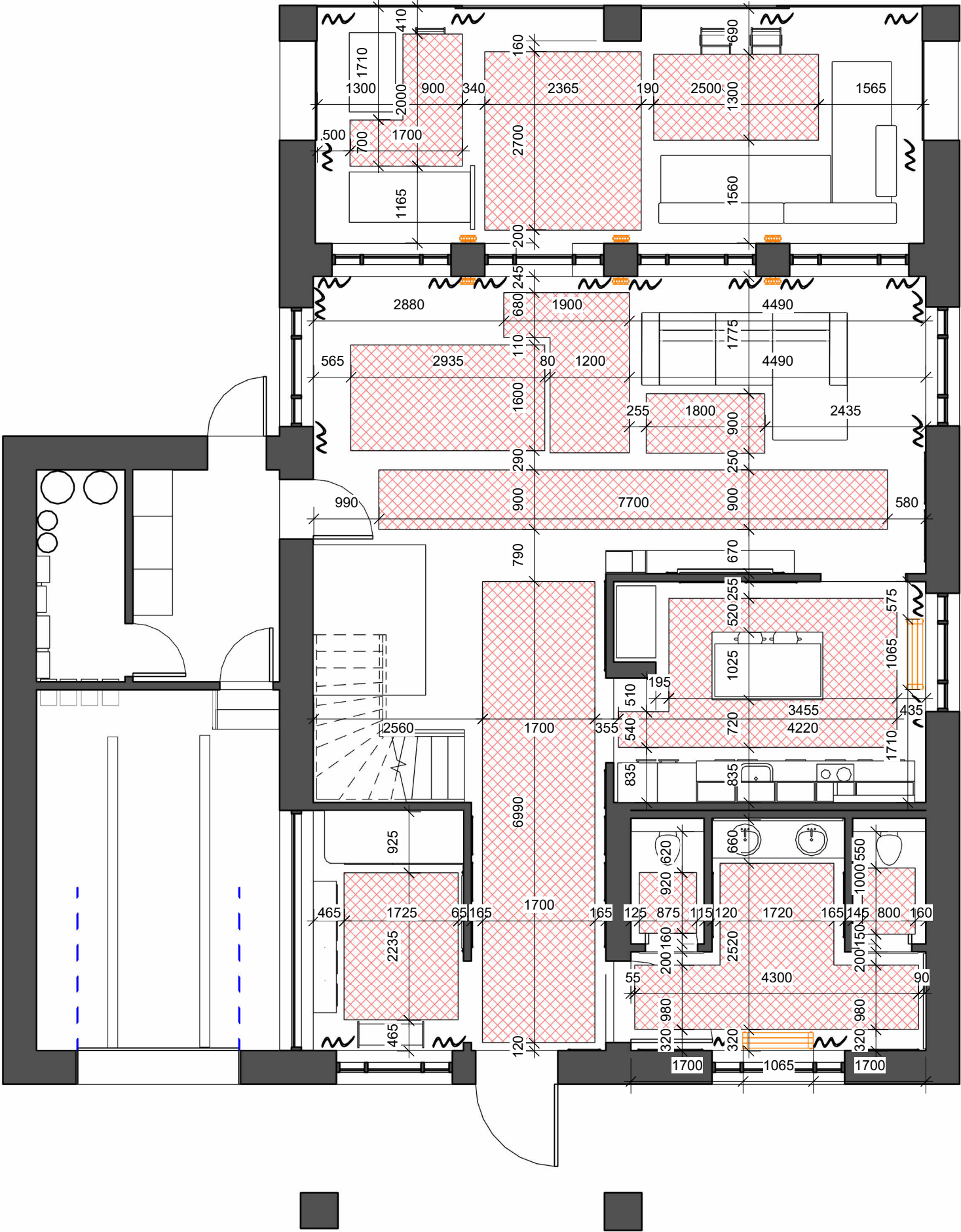
Level 1 План опалення
