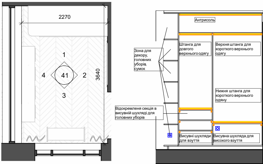
Level 1 Маркування Гардеробна
