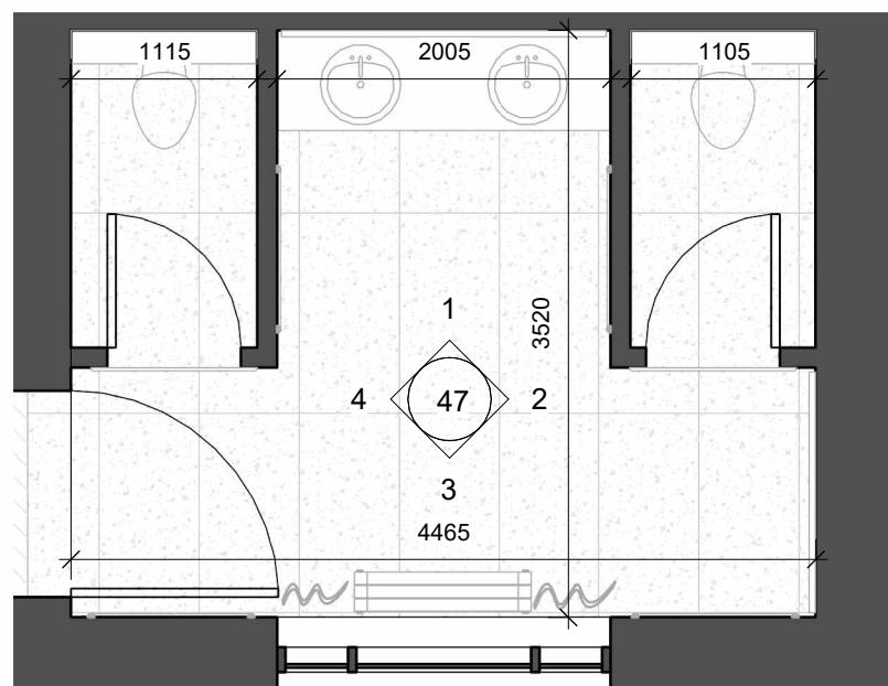
Level 1 Маркування Санвузол
