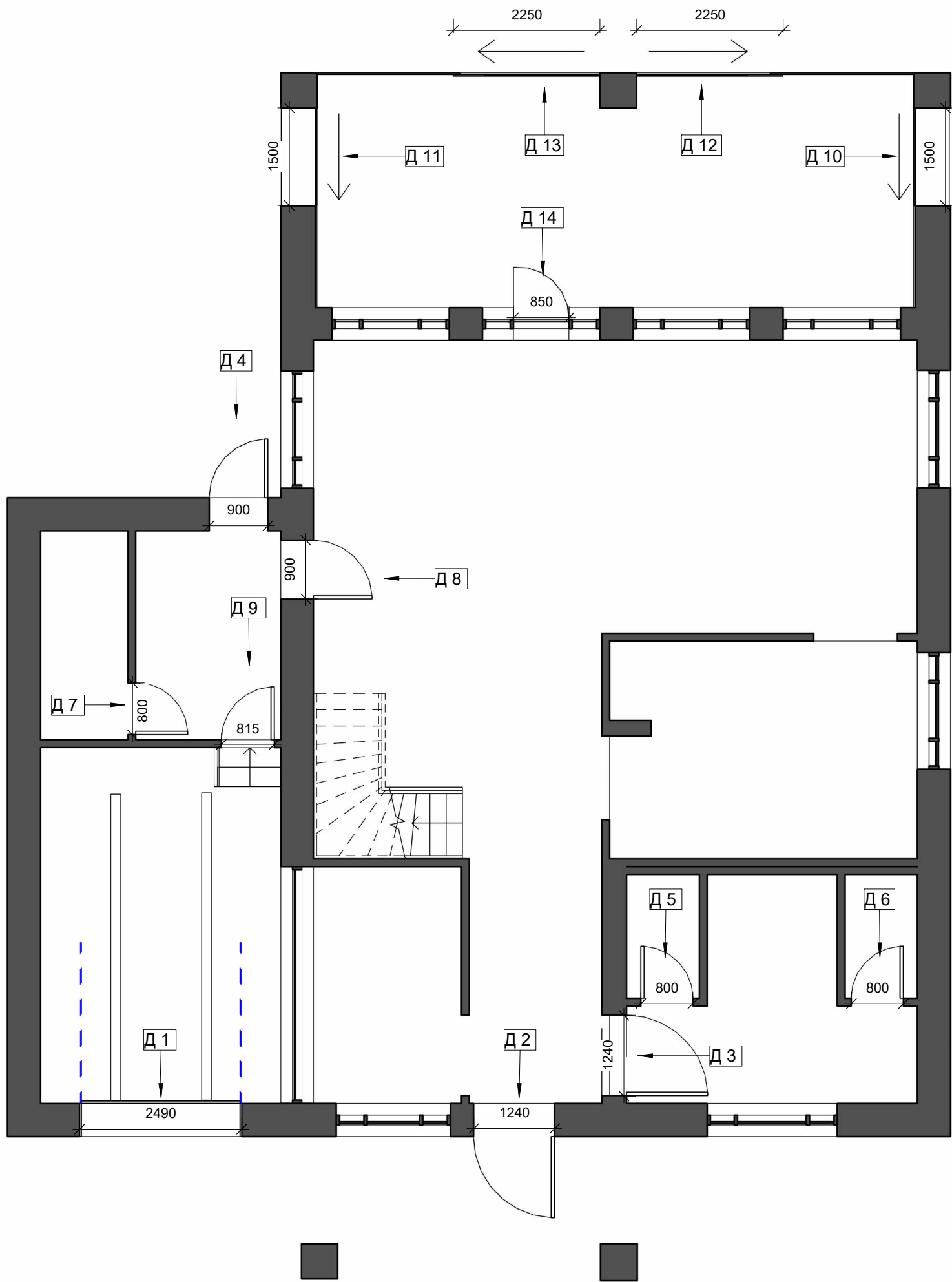
Level 1 План дверей
