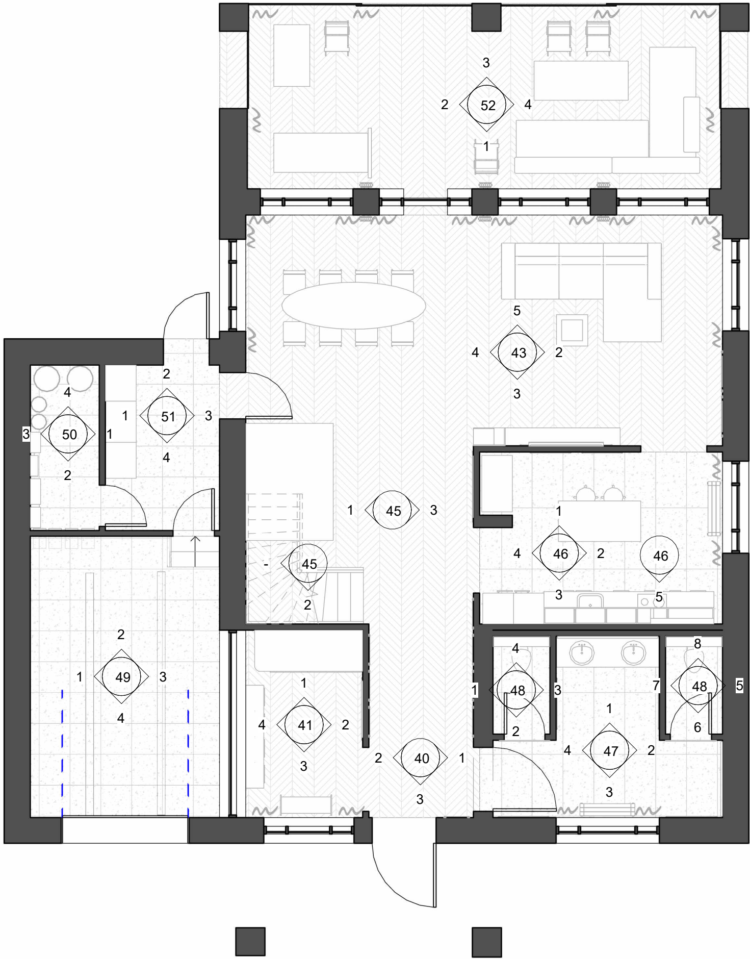
Level 1 Маркування кутів приміщень
