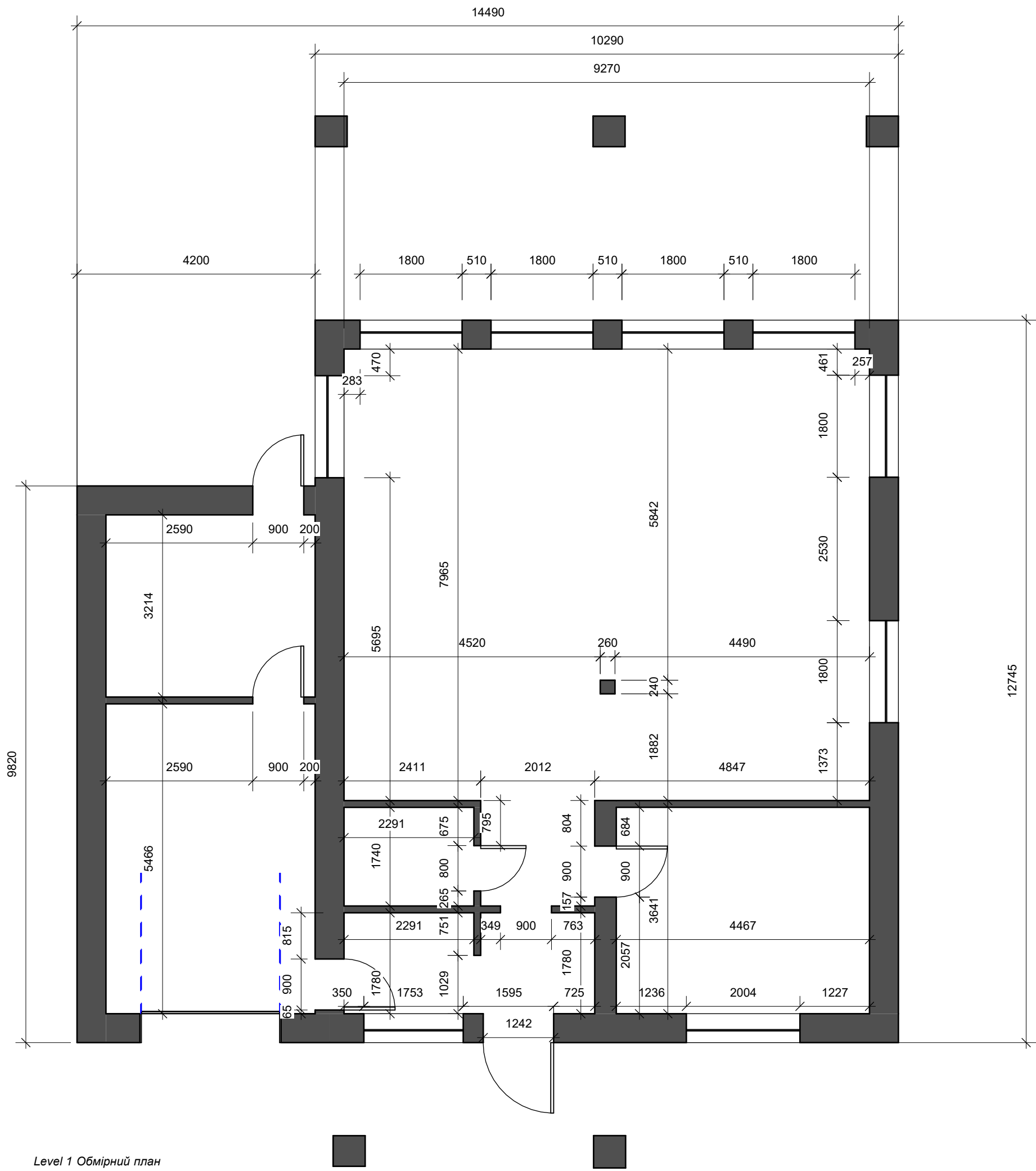
Level 1 Обмірний план
