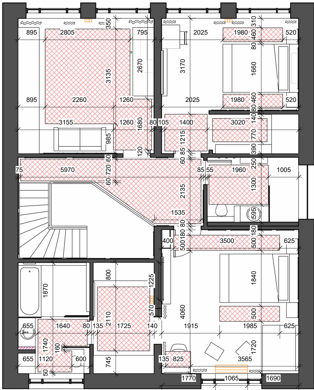
Level 2 План опалення
