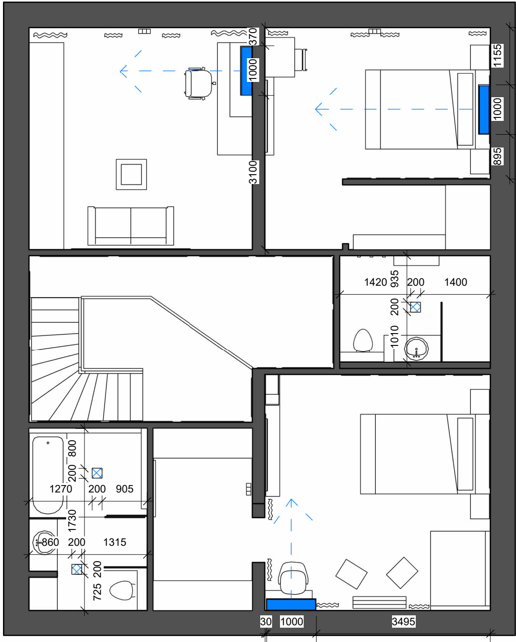
Level 2 План кондиювання
