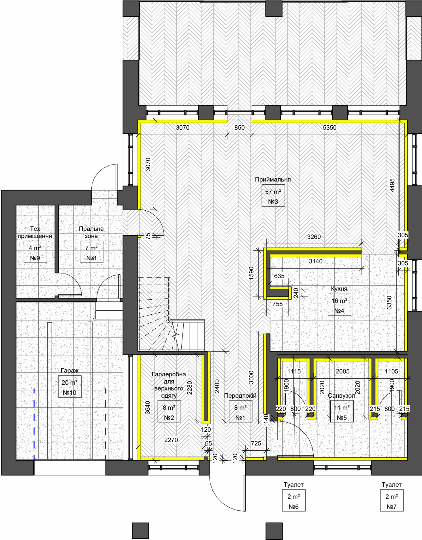
Level 1 План підлоги
