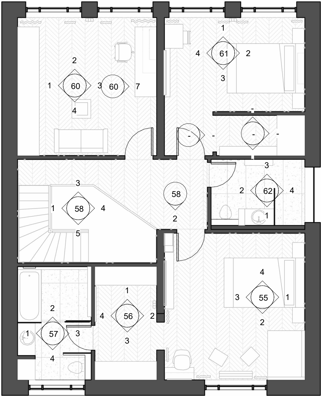
Level 2 Маркування кутів приміщень
