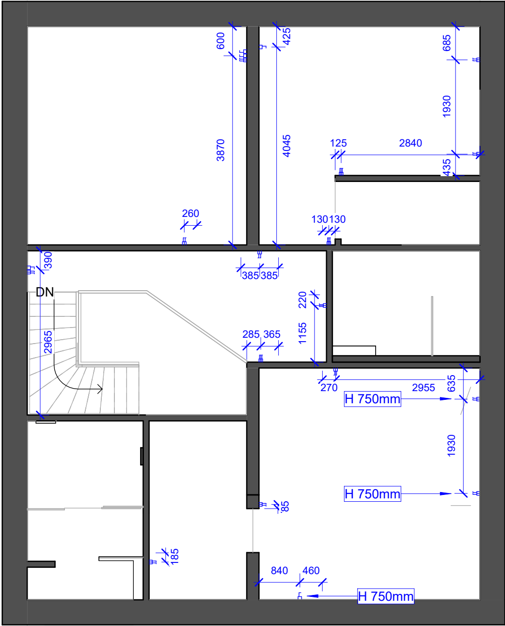
Level 2 Електрика перемикачі
