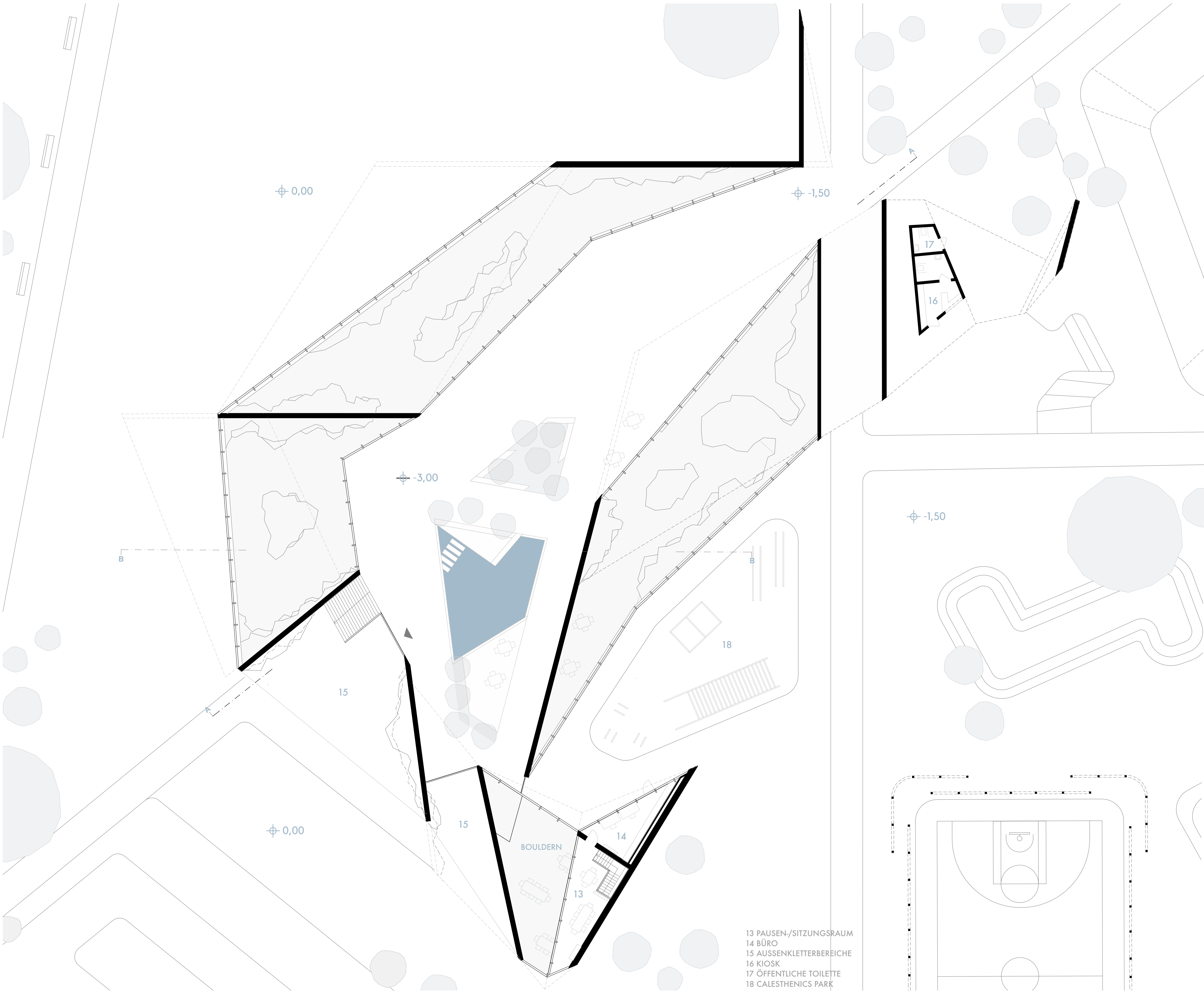
GRUNDRISS EG M 1:200
