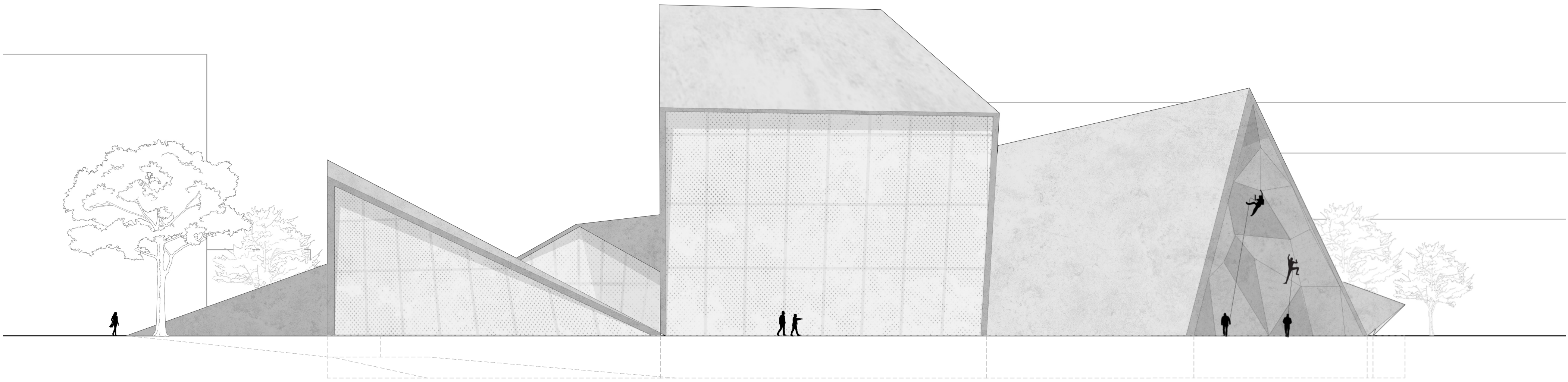
ANSICHT WEST M 1:200
