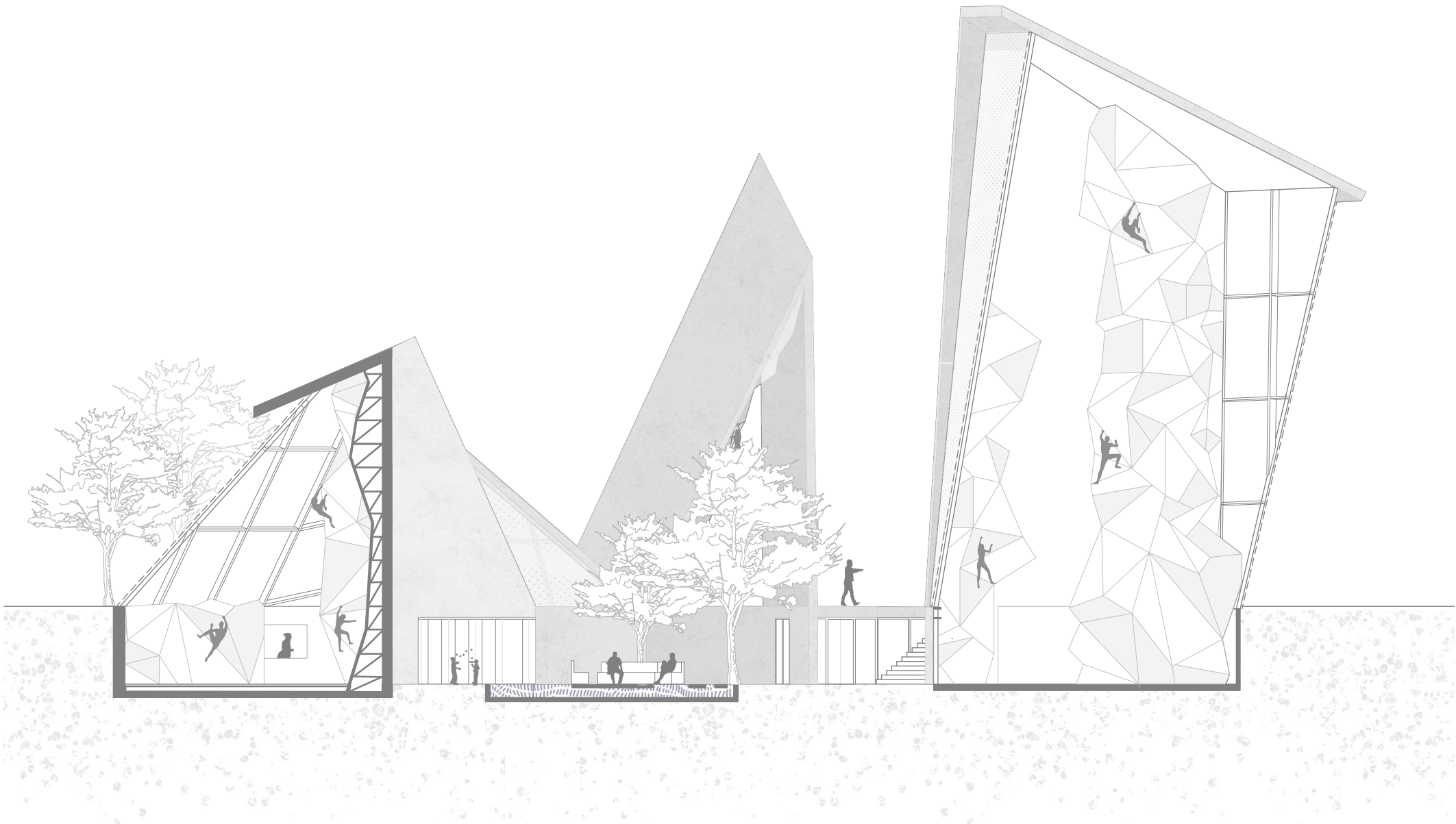
SCHNITT B-B M 1:200
