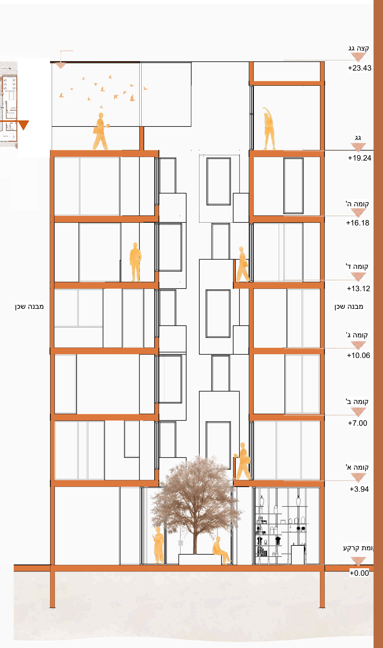
Section A-A
