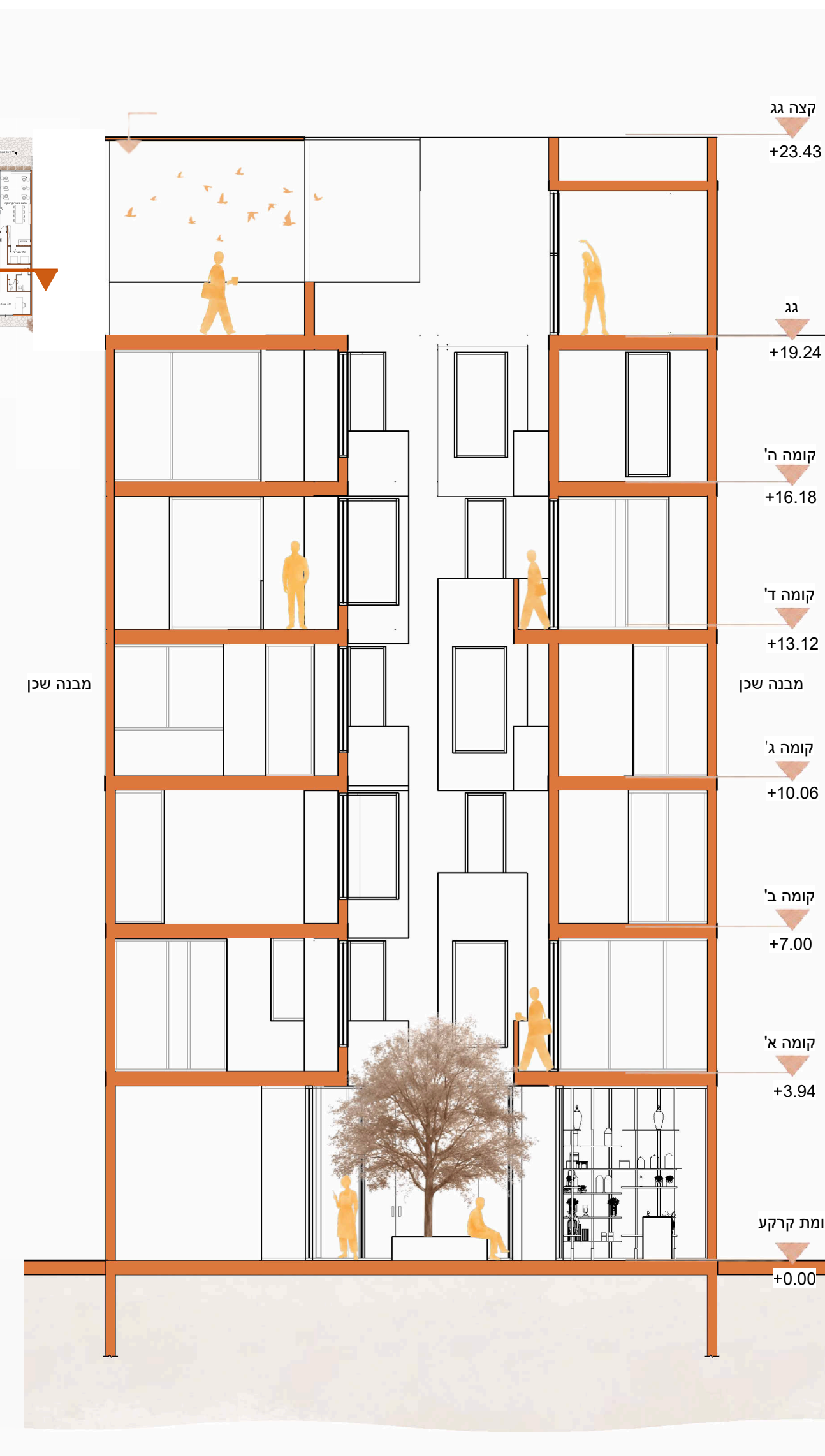
חתך א-א 1:00
