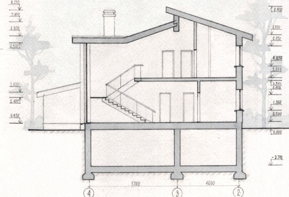
РОЗРІЗ ЧЕРЕЗ ВІСЬХ 4-2 А-А М 1:100 SECTION 4-2 A-A S 1:100
