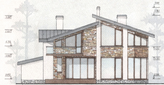
5 ФАСАД 5-1 М 1:100 FACADE 5-1 S 1:100
