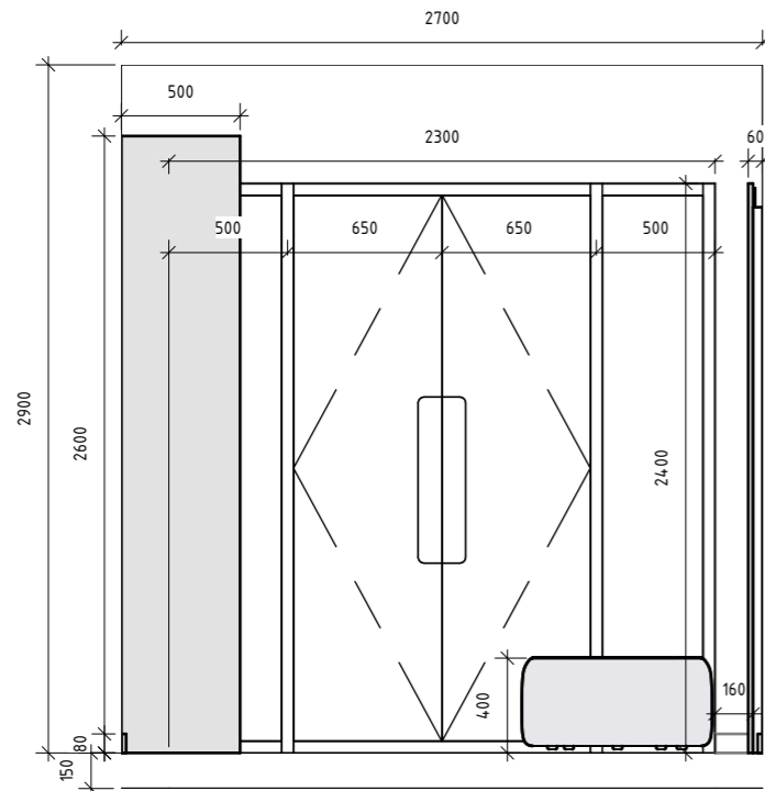
1 Передпокій А-В 1 : 35
