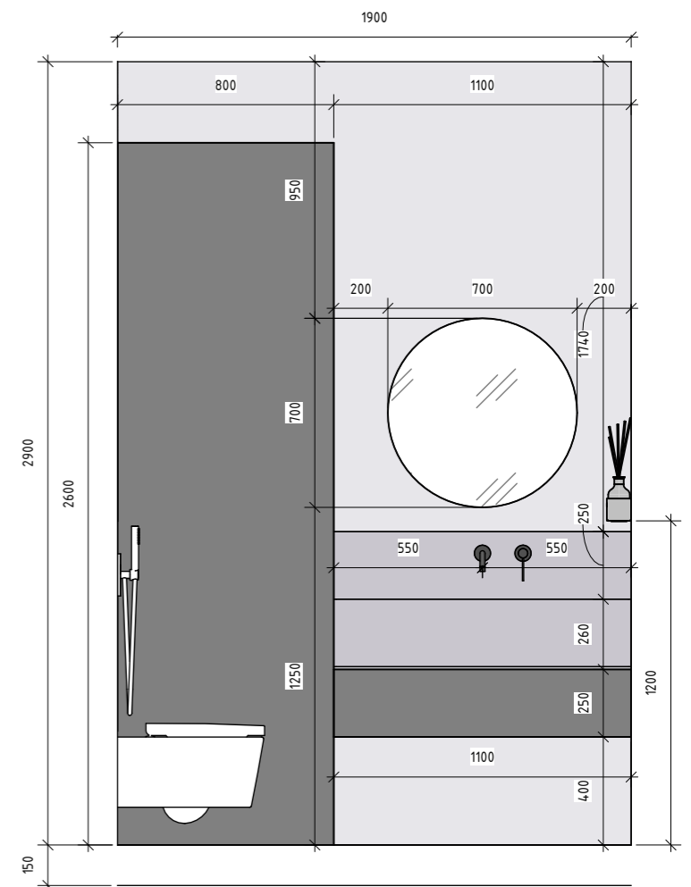
4 Санвузол Г-Б 1 : 25
