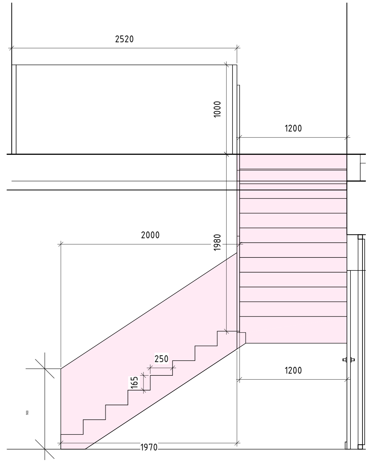
2 План сходів 1 : 25
