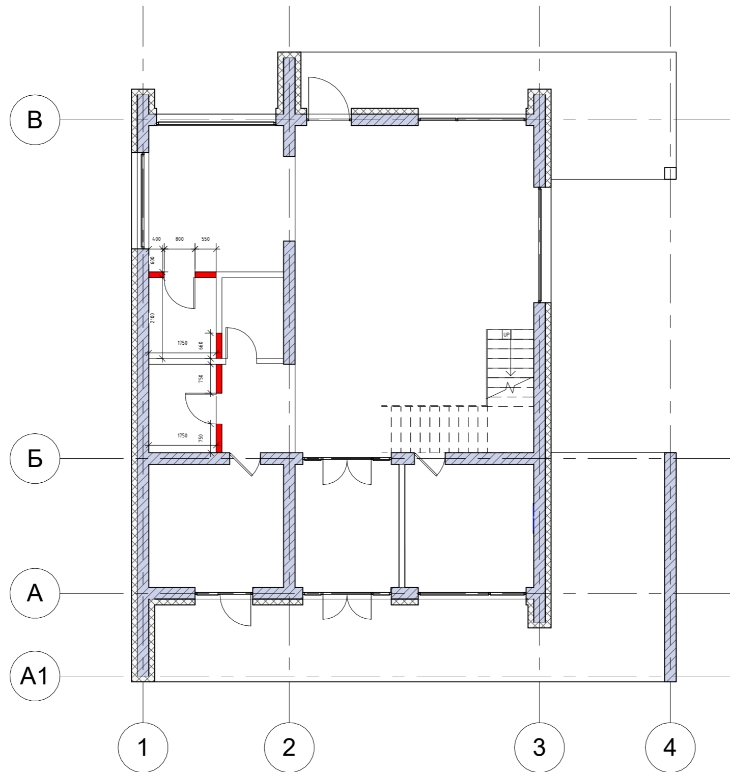
1 План демонтажу 1 поверх 1 : 100
