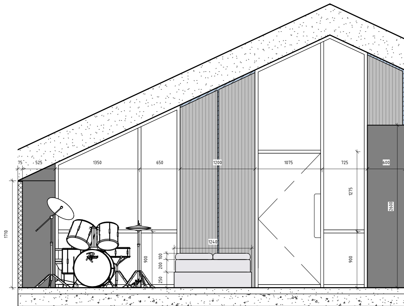
1 Спальня 2 А-Б 1 : 35
