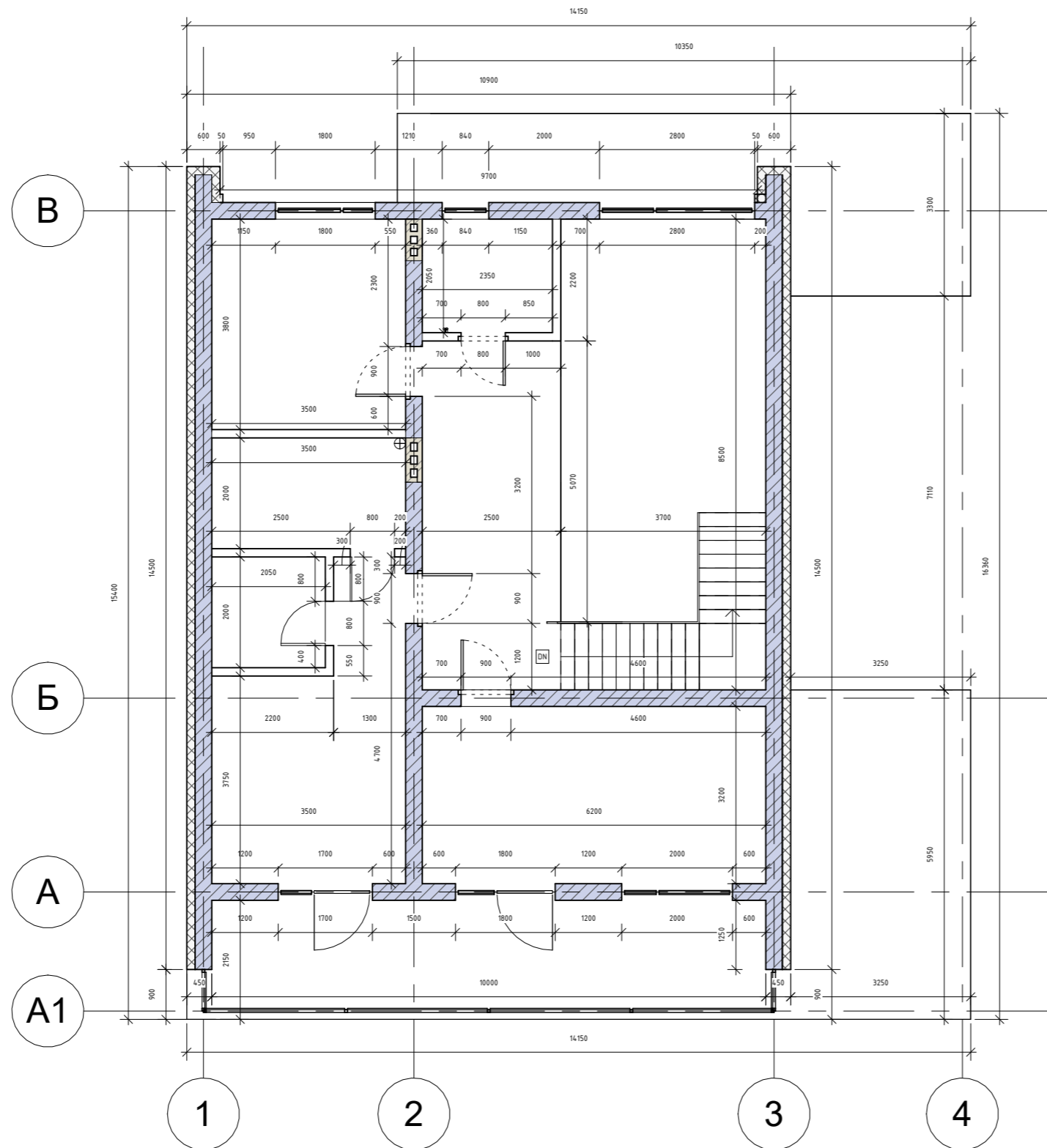
1 Вихідний план 2 поверх 1 : 100
