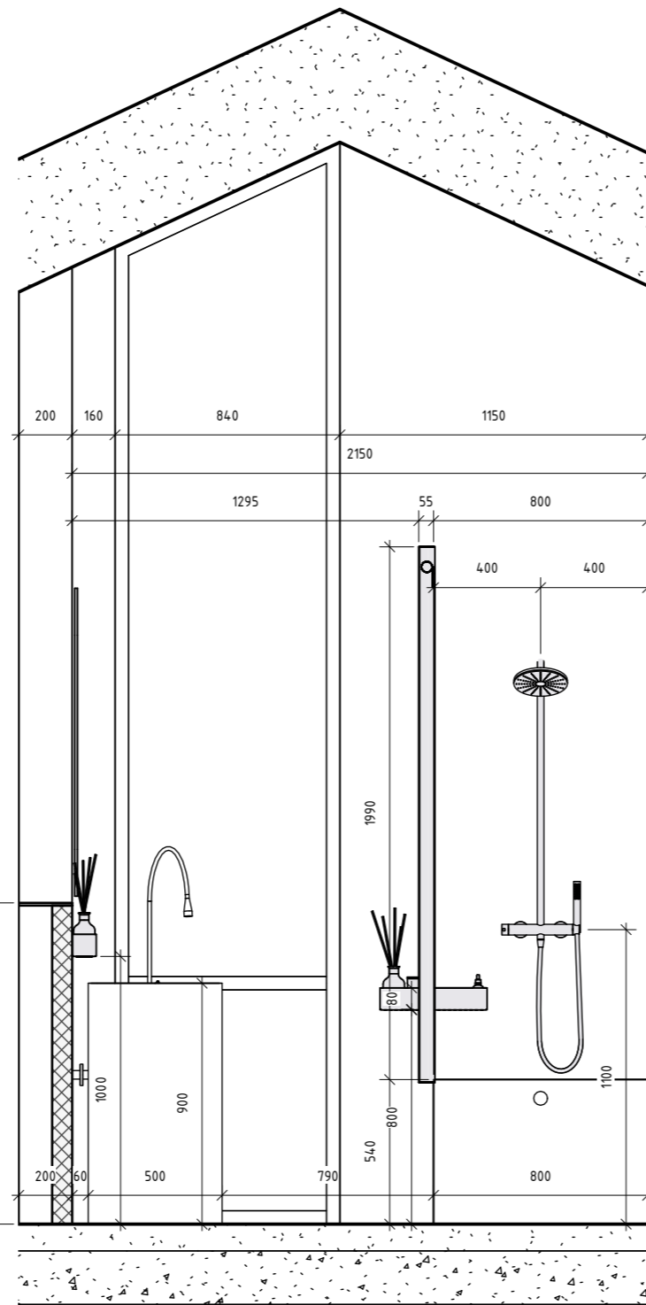
3 Санвузол 3 В-Г 1 : 25
