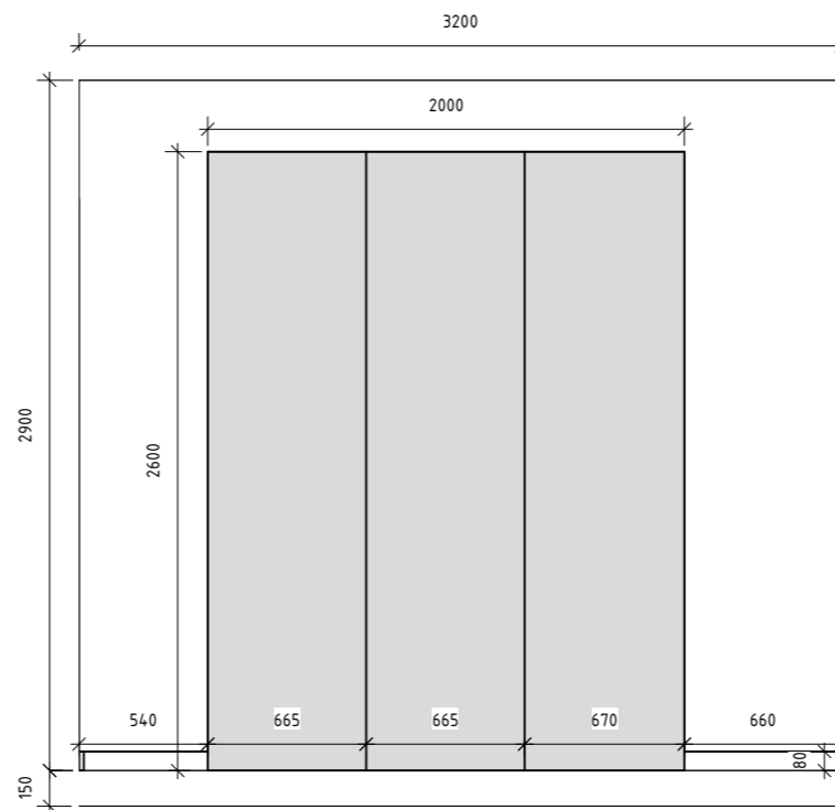
4 Передпокій Г-Б 1 : 35
