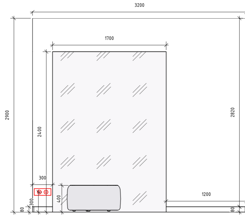
2 Передпокій А-В 1 : 35
