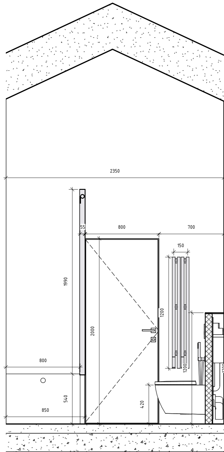
1 Санвузол 3 А-Б 1 : 25
