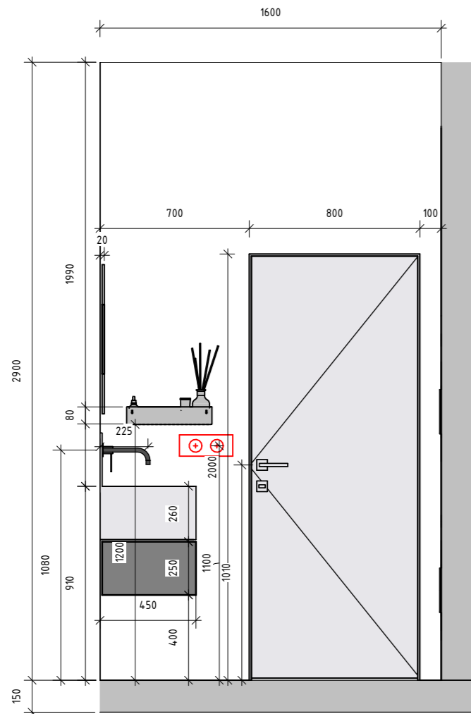
1 Санвузол А-Б 1 : 25
