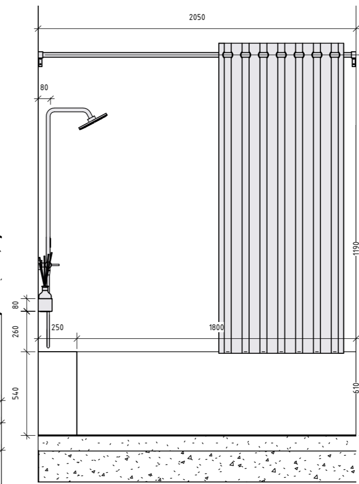
4 Санвузол 3 Г-Б 1 : 25
