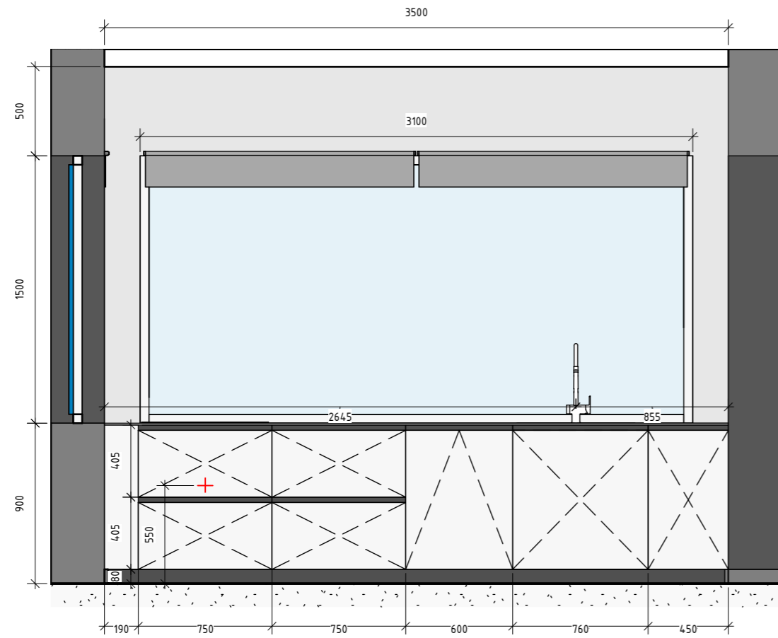
1 Розгортки кухні 1 : 30
