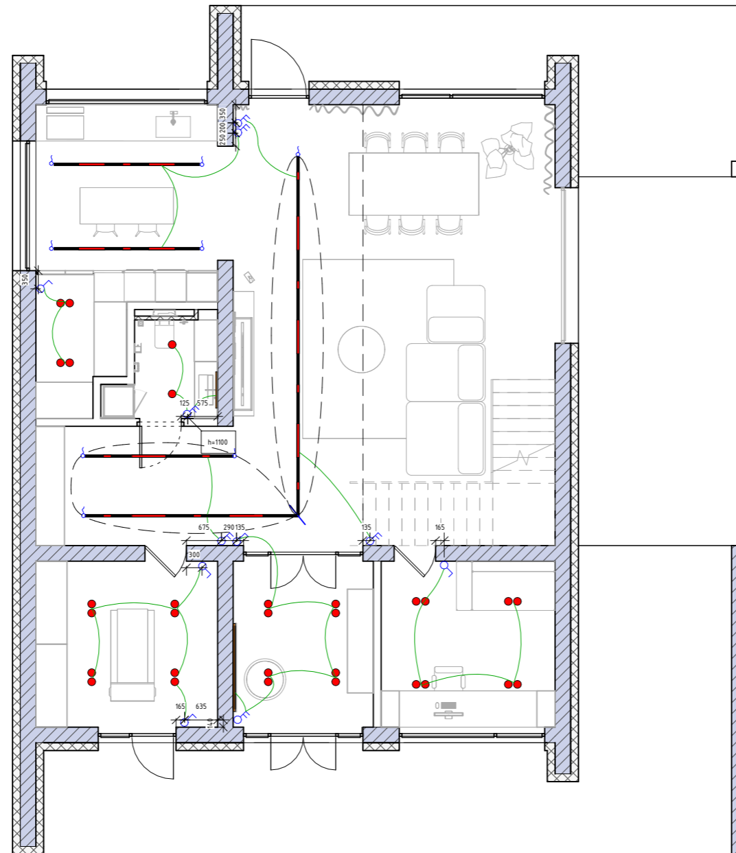
1 План вимикачів 1 поверх 1 : 100
