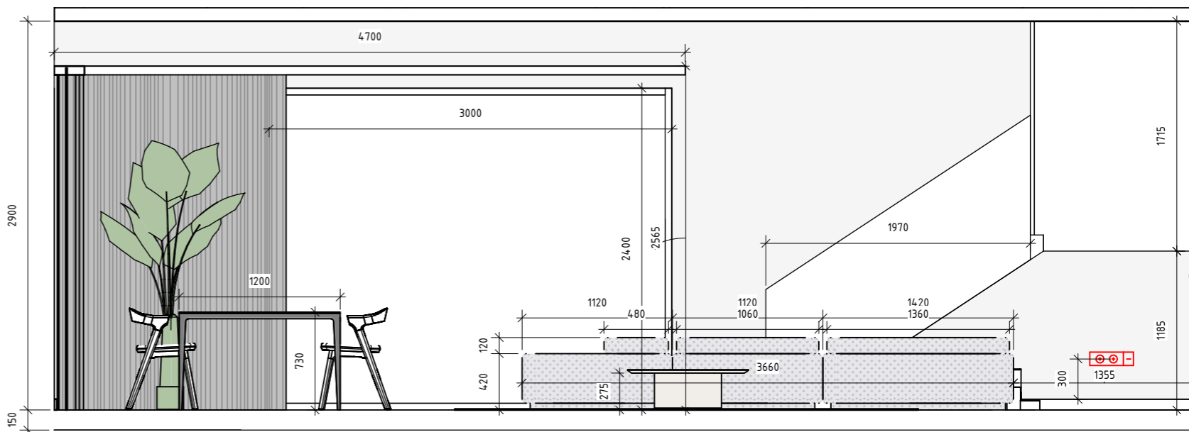
4 Вітальня Г-Б 1 : 40
