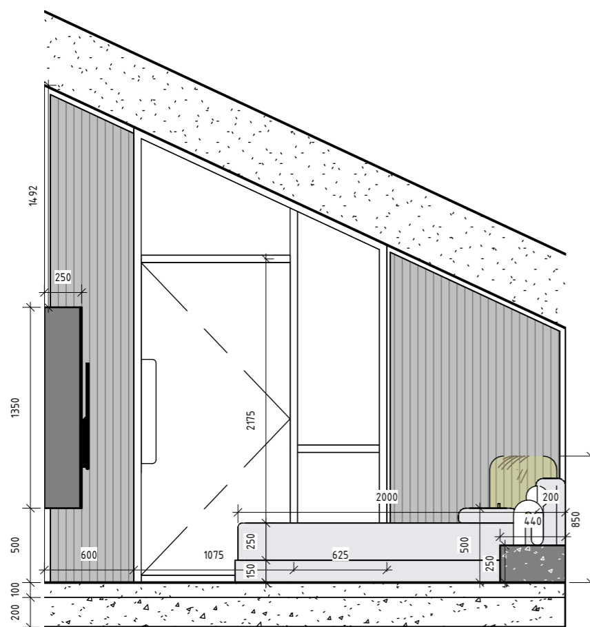
3 Майстер спальня А-Б 1 : 35
