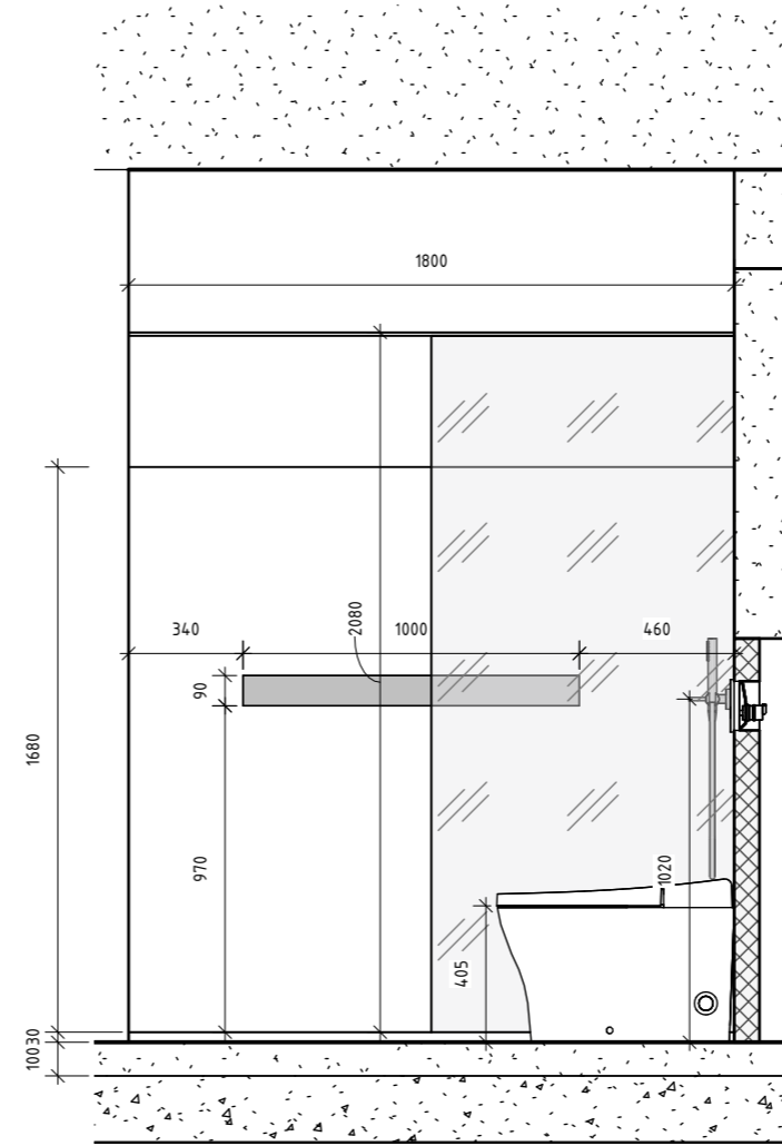
2 Майстер санвузол А-В 1 : 25
