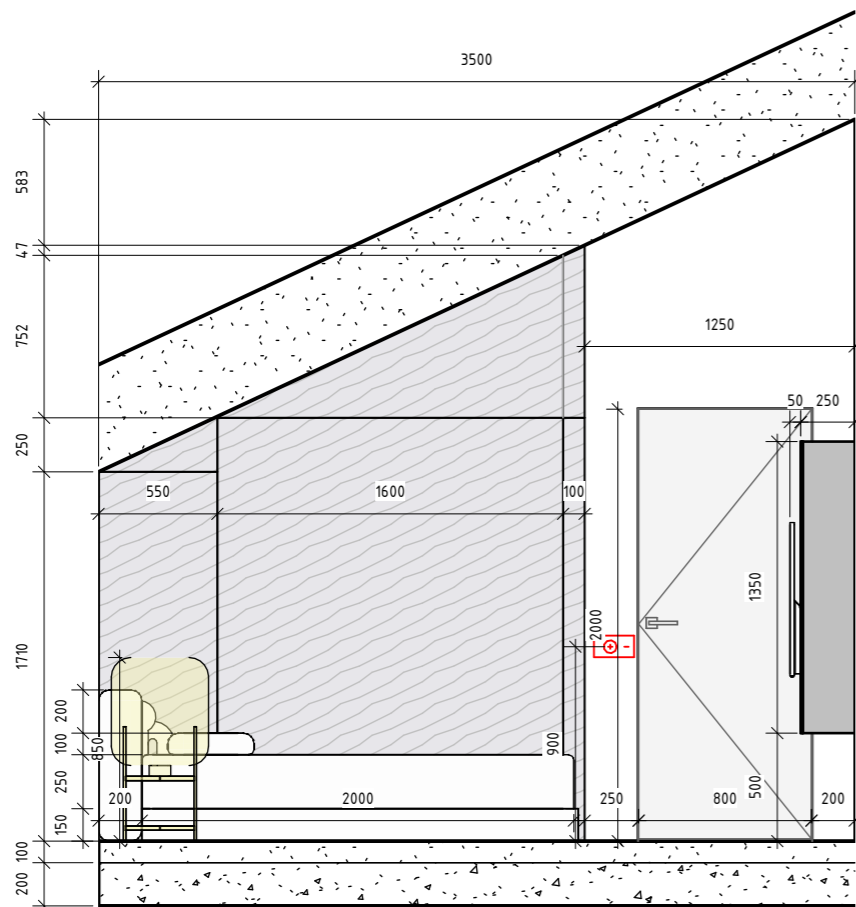
1 Майстер спальня В-Г 1 : 35
