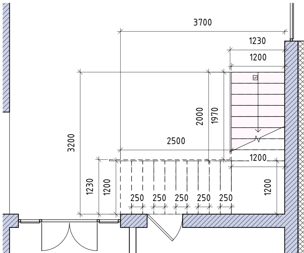
1 План сходів 1 : 50
