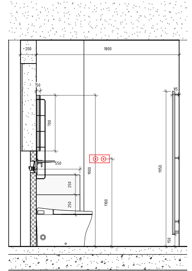
4 Майстер санвузол Г-Б 1 : 25
