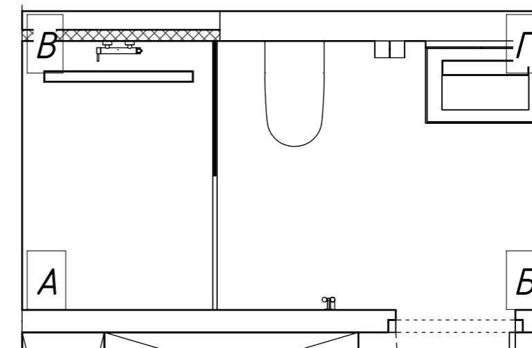
2 Майстер санвузол А-В 1 : 25
