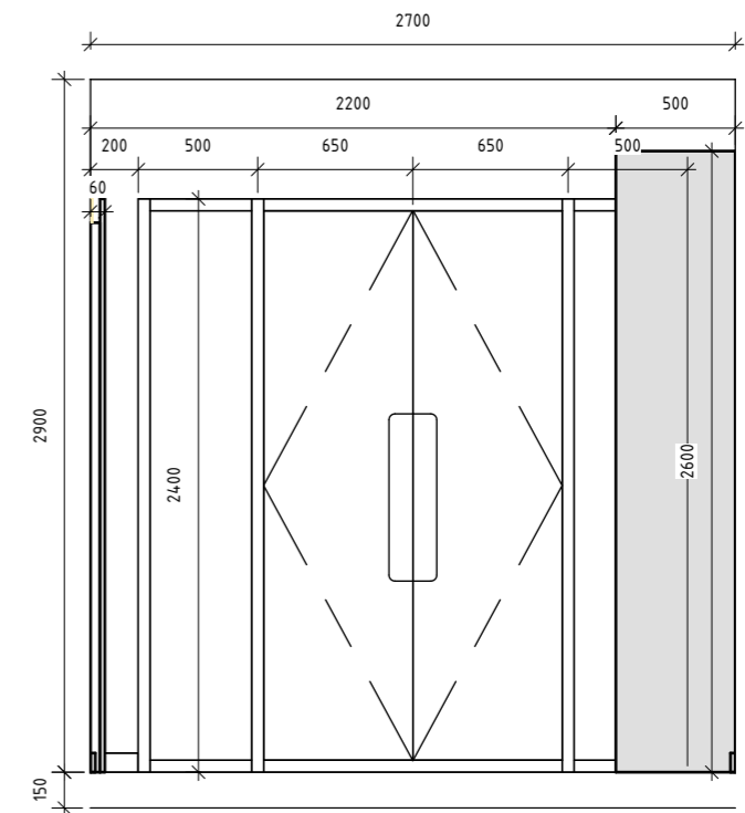
3 Передпокій В-Г 1 : 35
