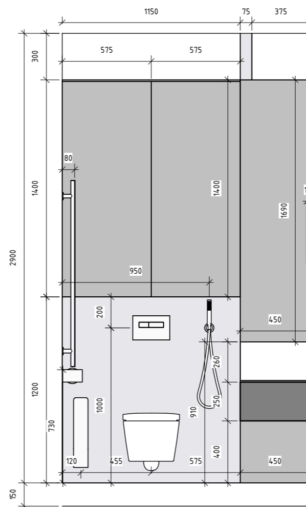
3 Санвузол В-Г 1 : 25
