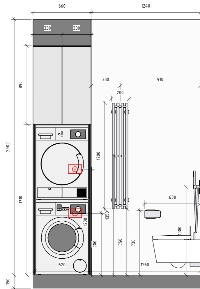
2 Санвузол А-В 1 : 25
