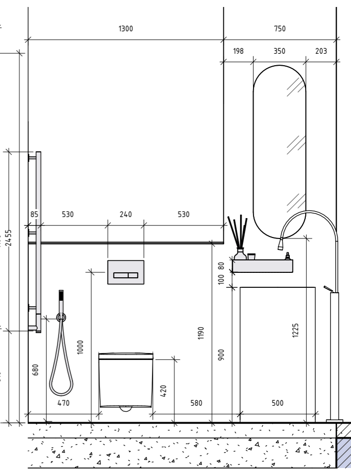
2 Санвузол 3 А-В 1 : 25
