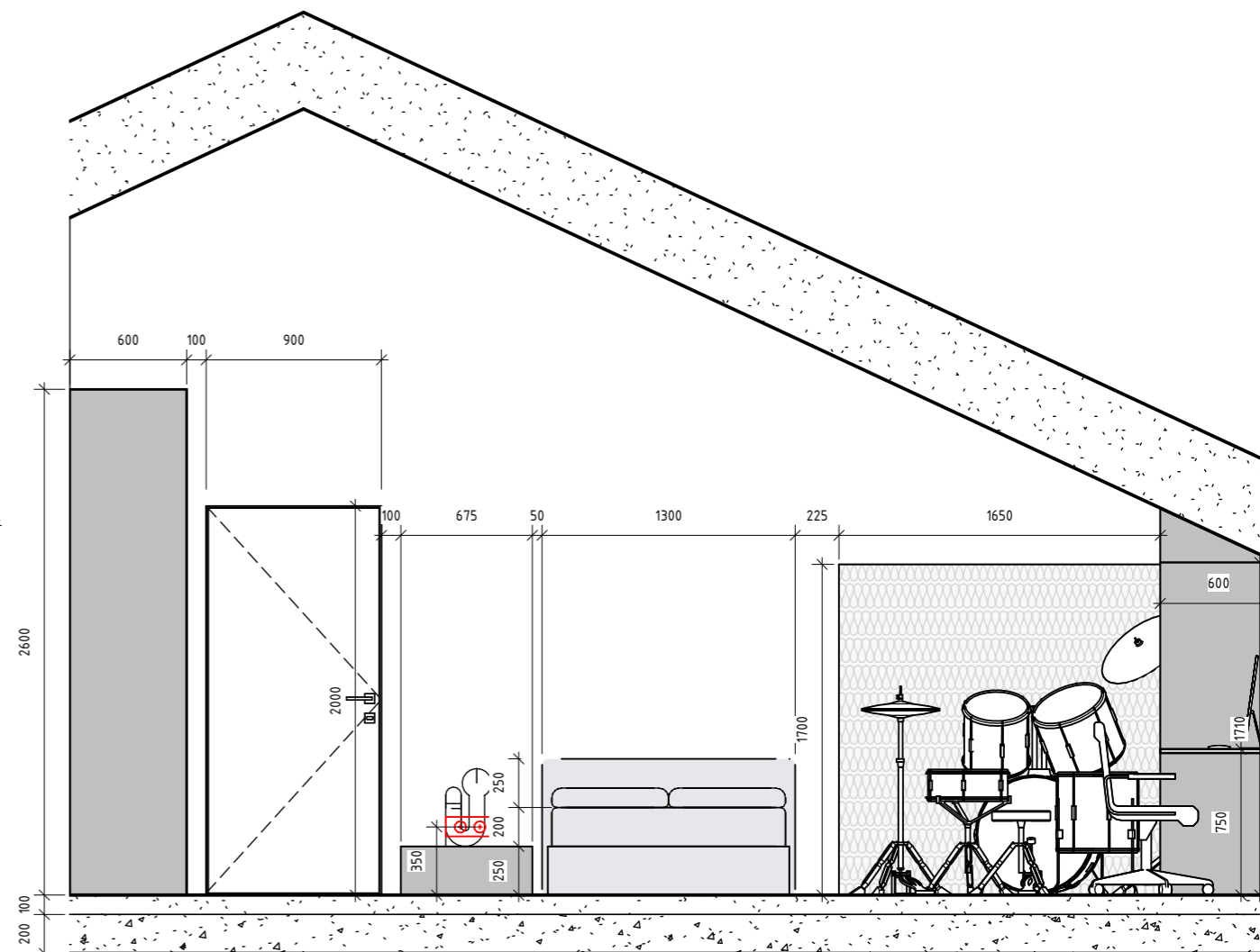
3 Спальня 2 В-Г 1 : 35
