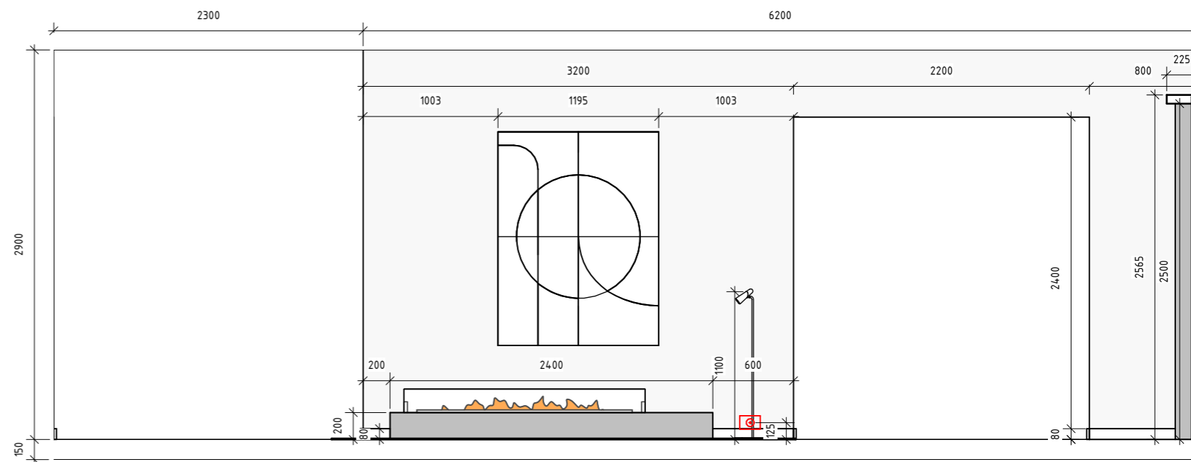
2 Вітальня А-В 1 : 40
