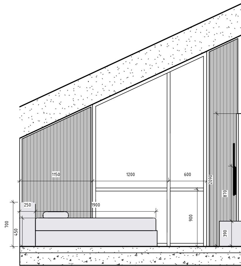
1 Спальня 3 В-Г 1 : 35
