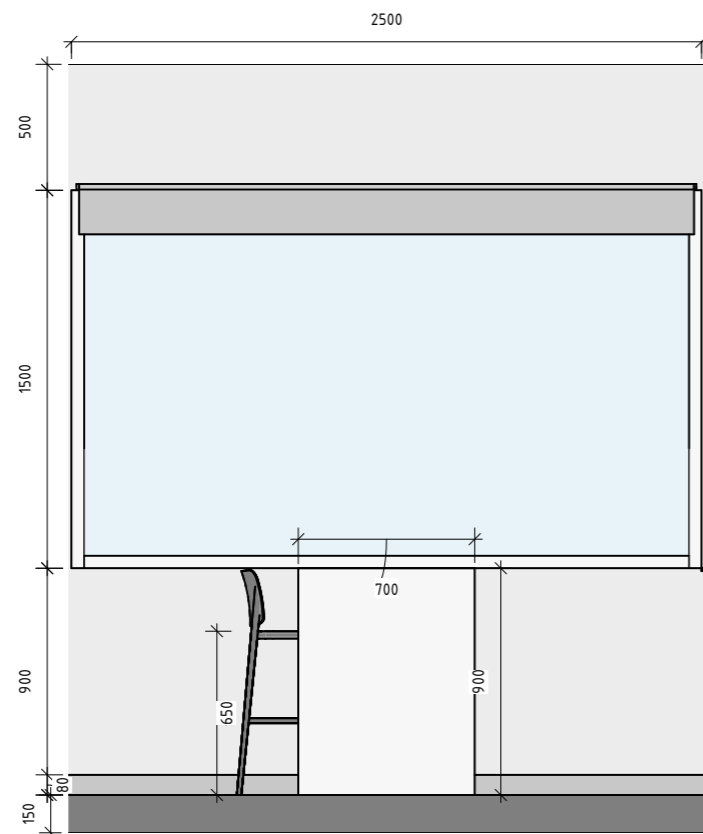
3 Розгортка острова бокова 1 : 30
