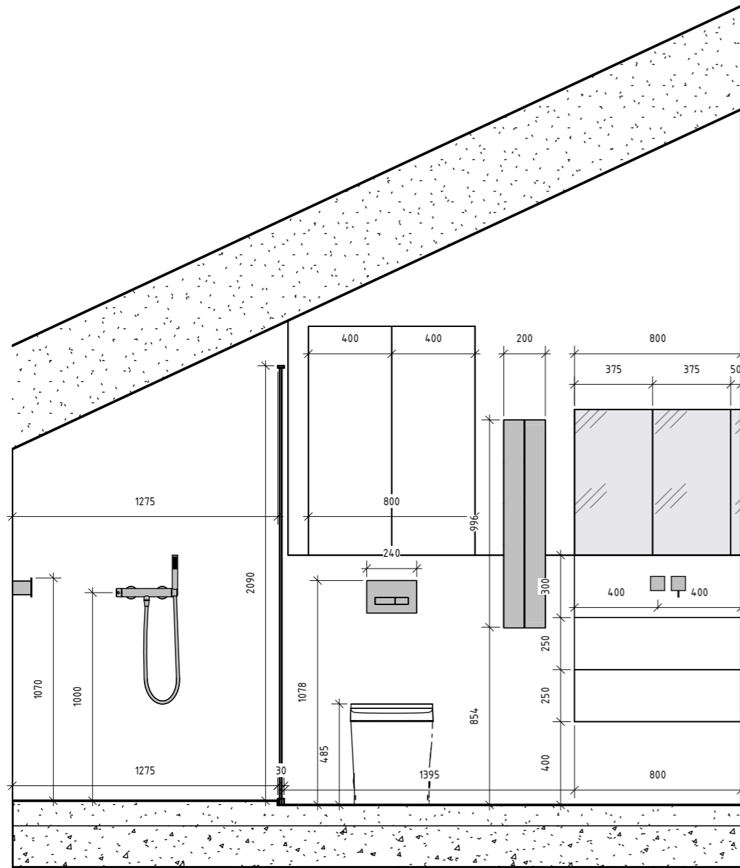
3 Майстер санвузол В-Г 1 : 25
