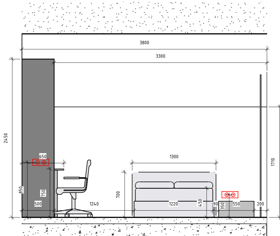
2 Спальня 3 А-В 1 : 35
