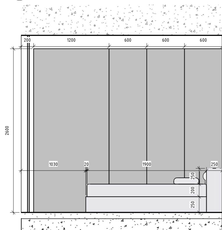
2 Спальня 2 А-В 1 : 35
