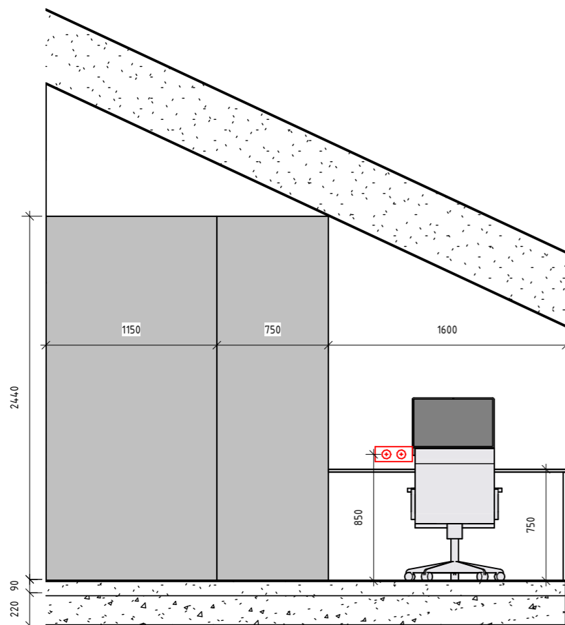
3 Спальня 3 А-Б 1 : 35
