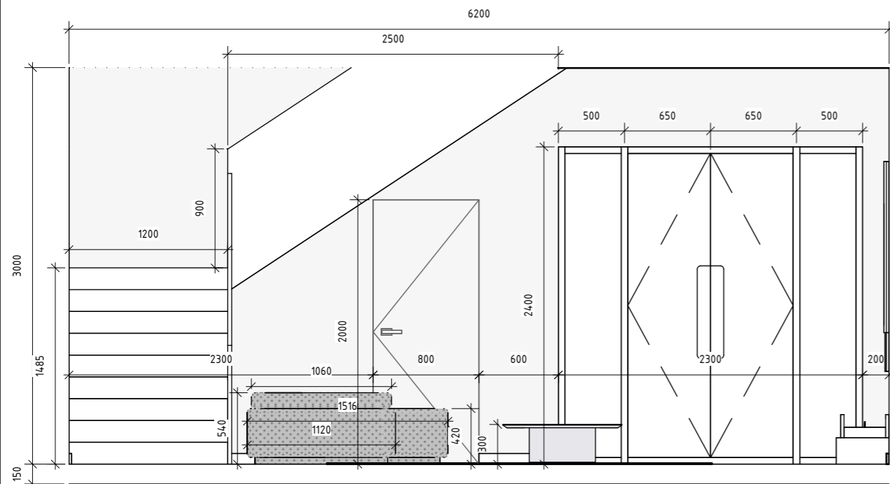
1 Вітальня А-Б 1 : 40
