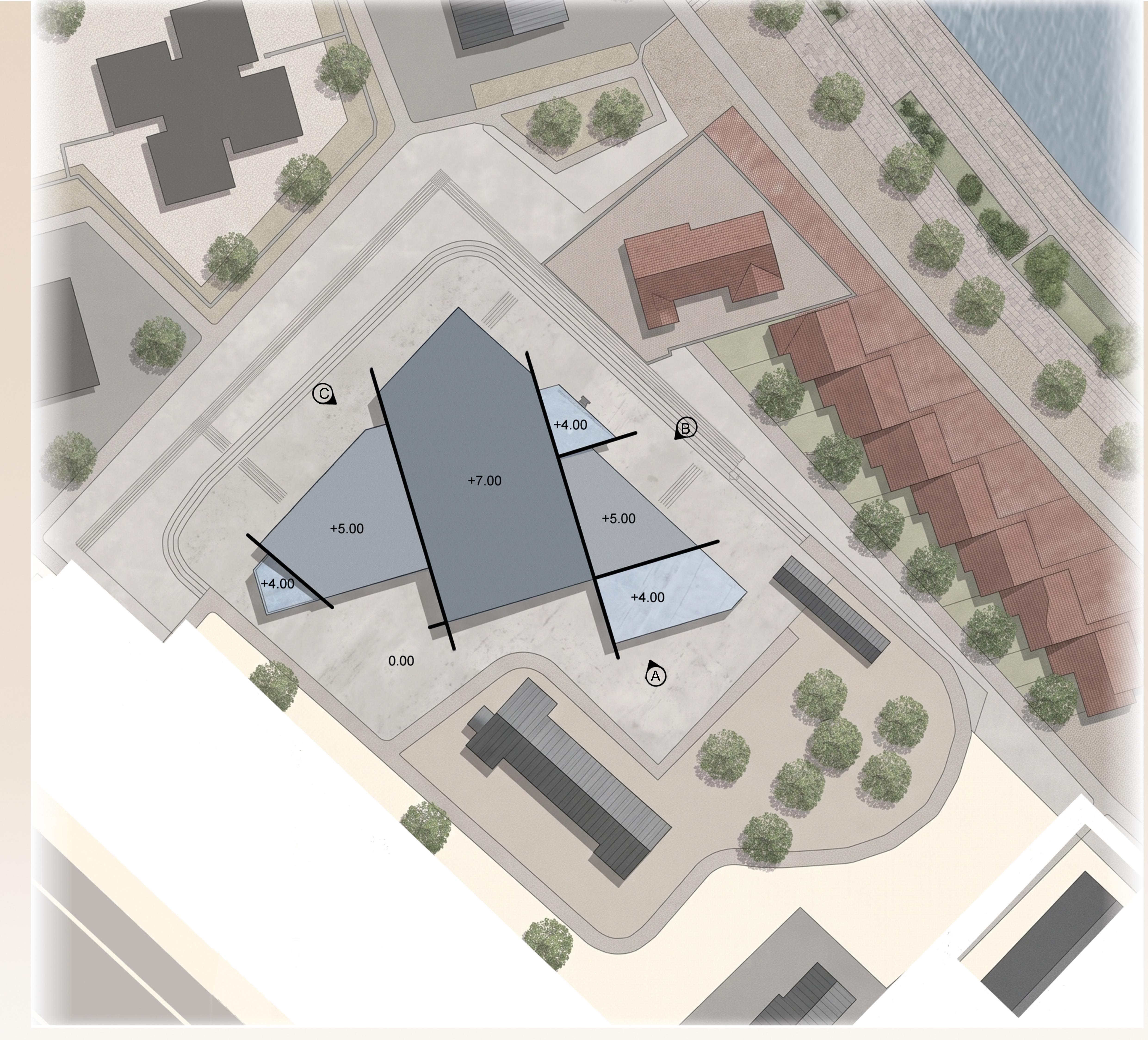
SITE PLAN 1:500
