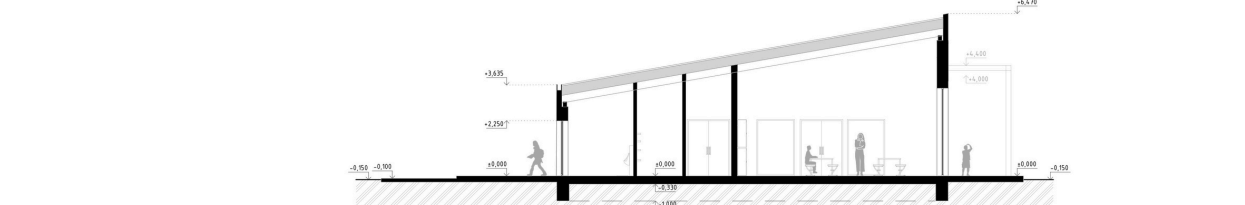
REZ D-D'
