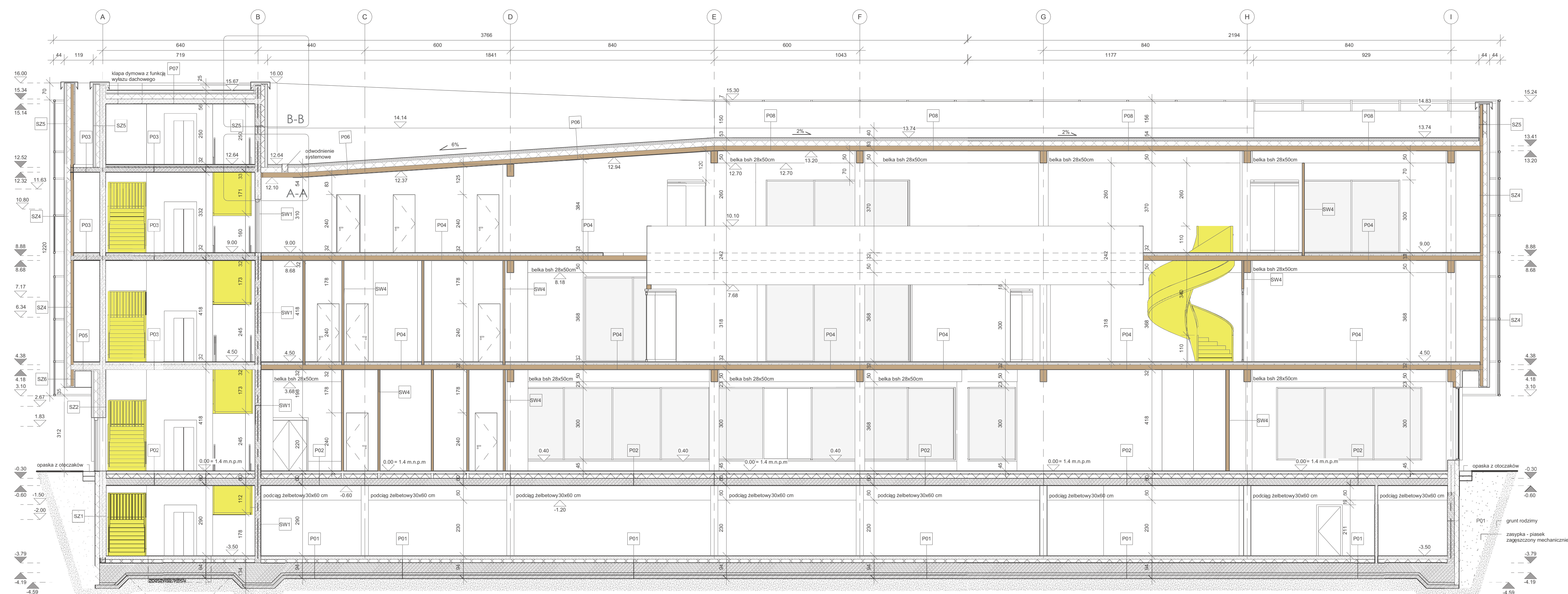
PRZEKRÓJ A-A SKALA 1:100
