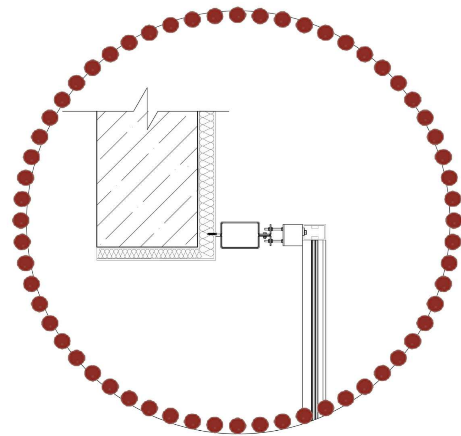
MESH BİRLEŞİM DETAYI - 1/5
