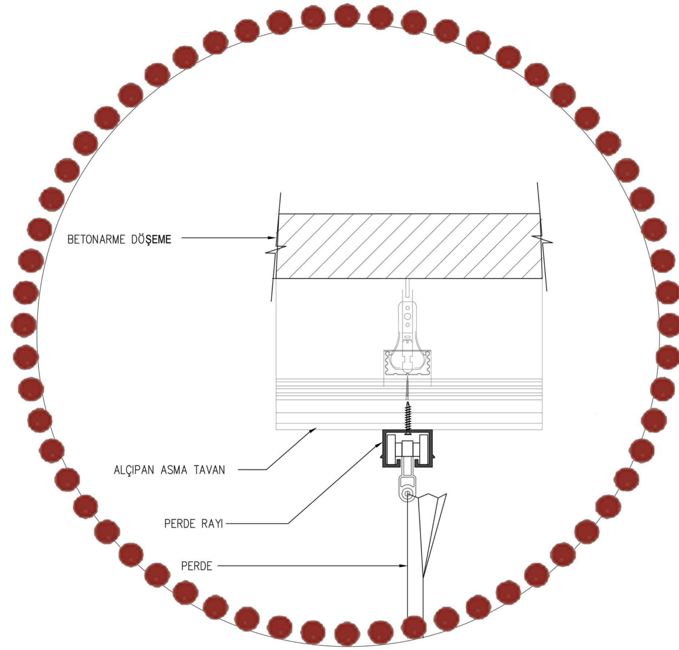
PERDE RAY DETAYI -1/5
