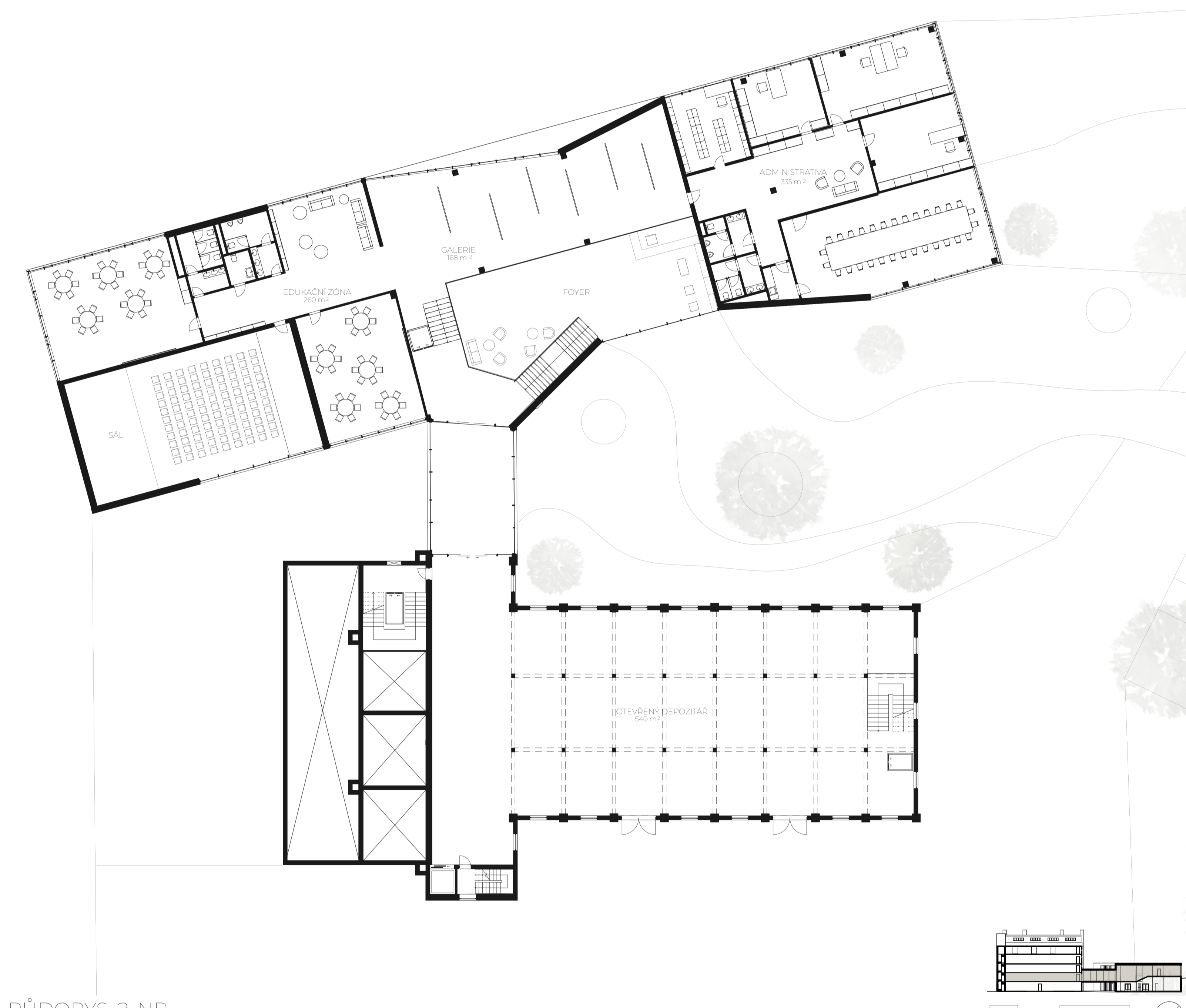
PŮDORYS 2. NP
