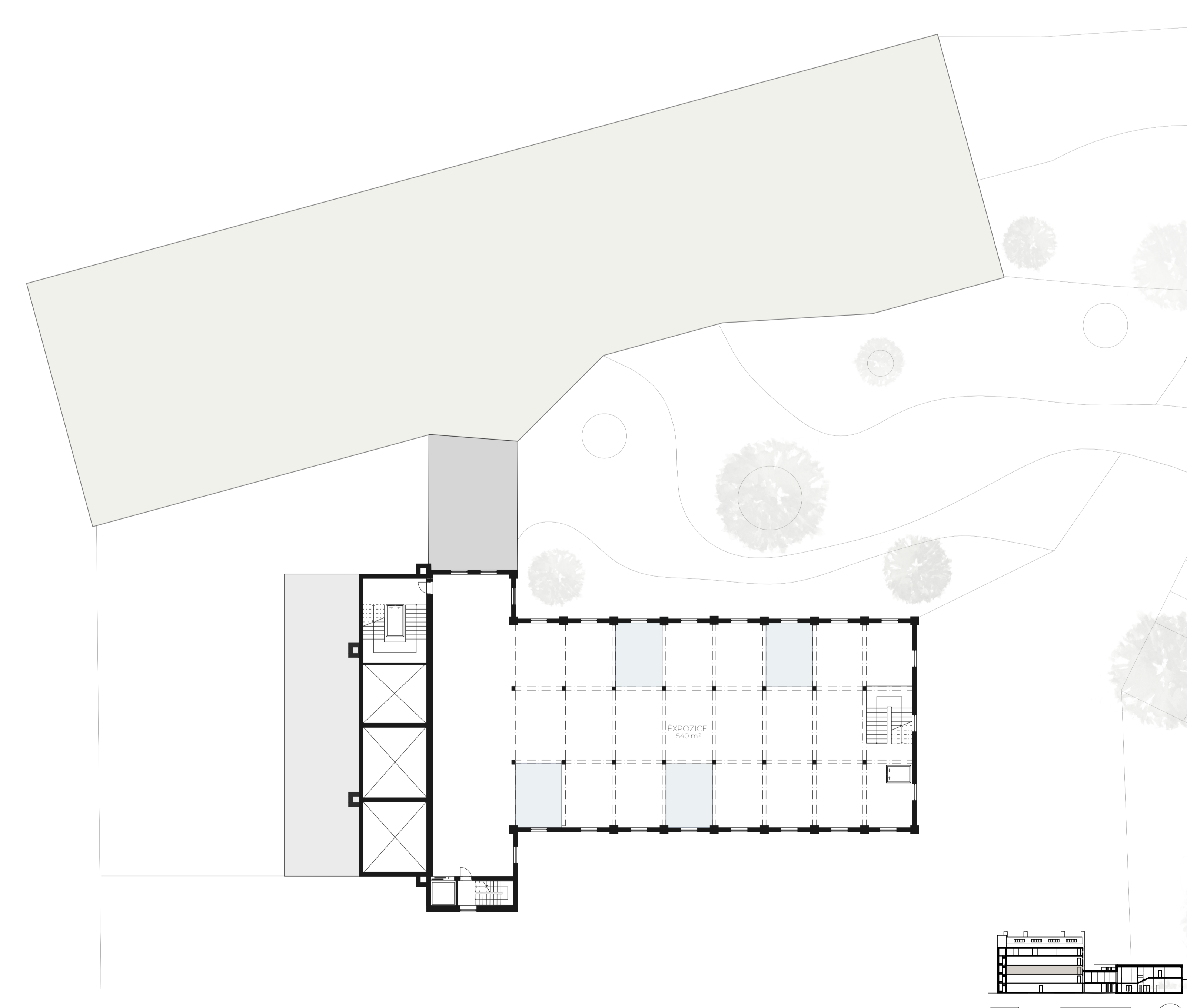
PŮDORYS 3. NP
