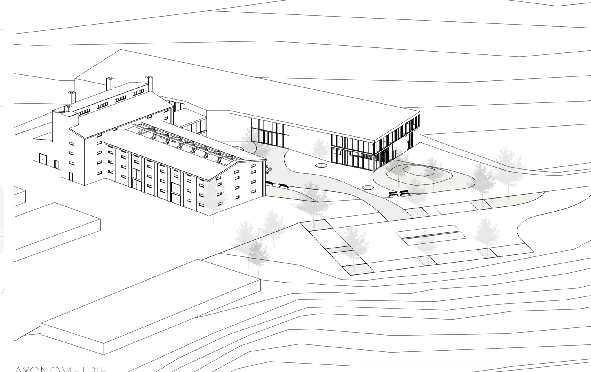
AXONOMETRIE
