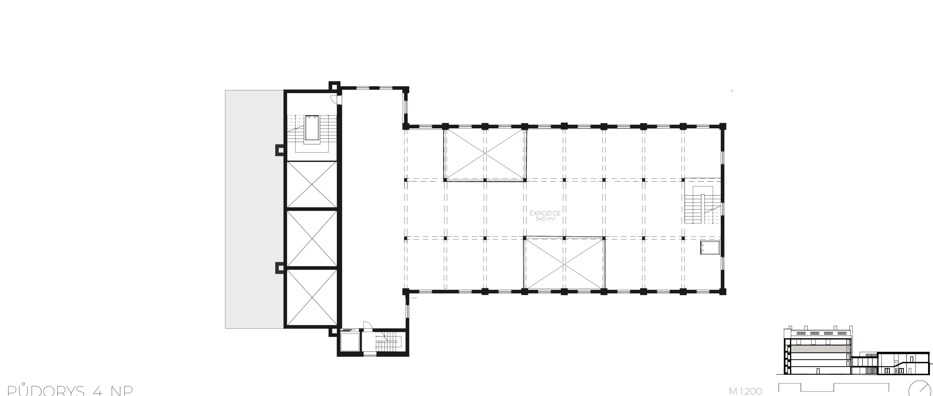
PŮDORYS 4. NP
