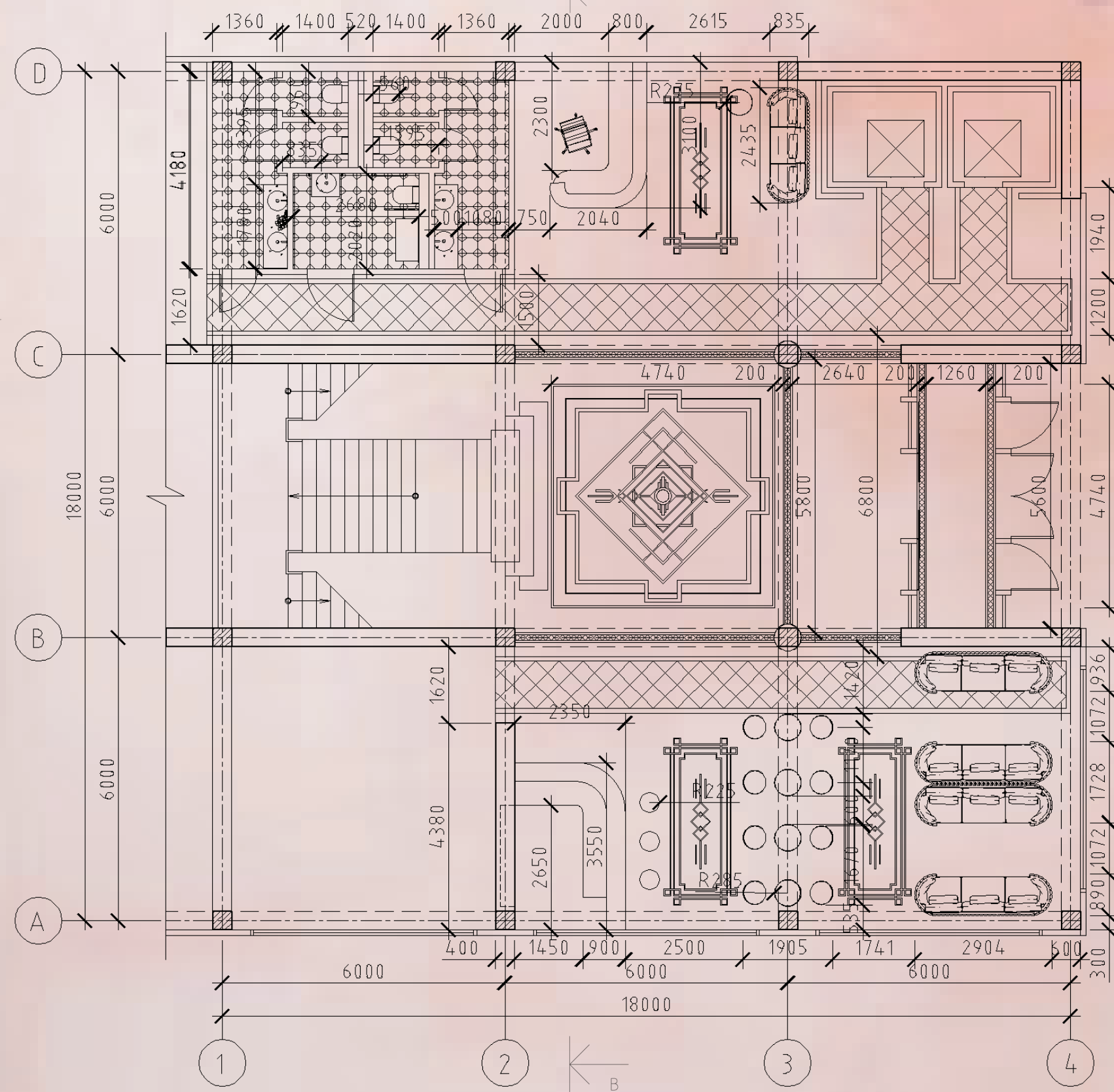
PLAN AMPLASARE
