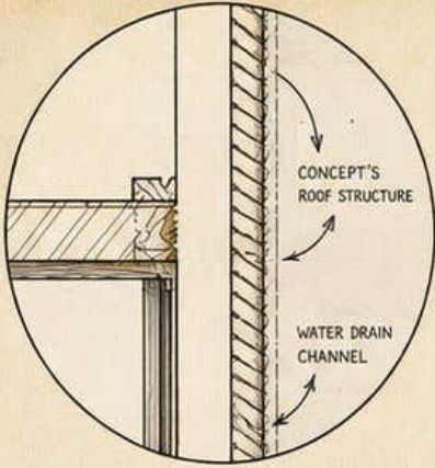
DETAIL A ROOF EDGE
