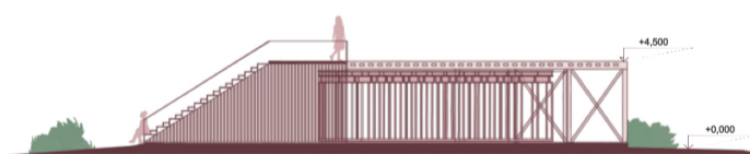
POHLED 1:100
