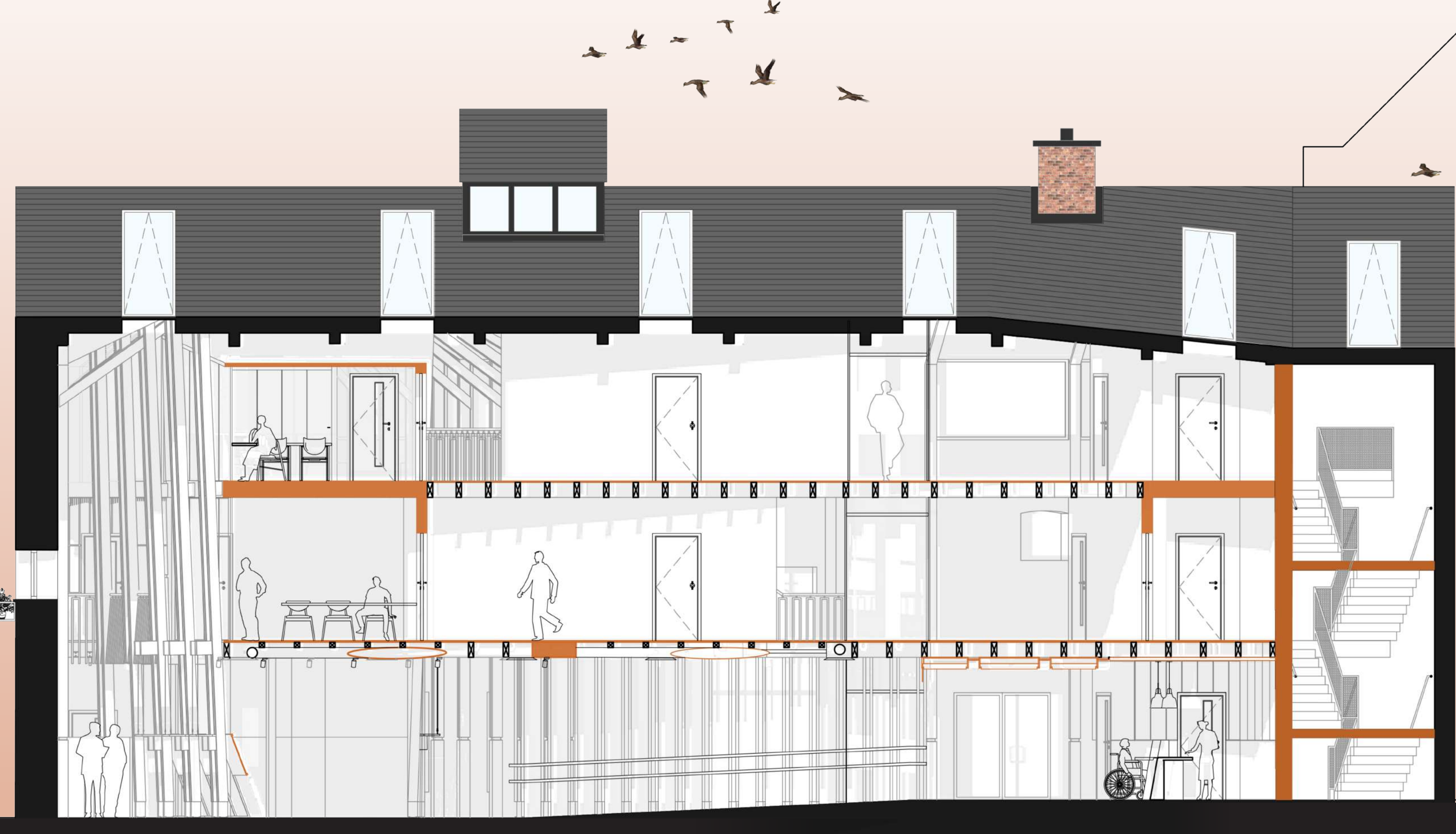
SECTION B.B
