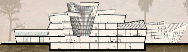
قطاع C-C
