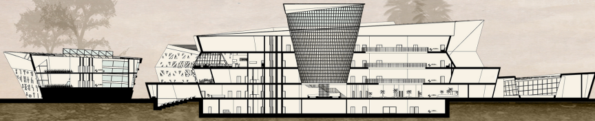
قطاع A-A
