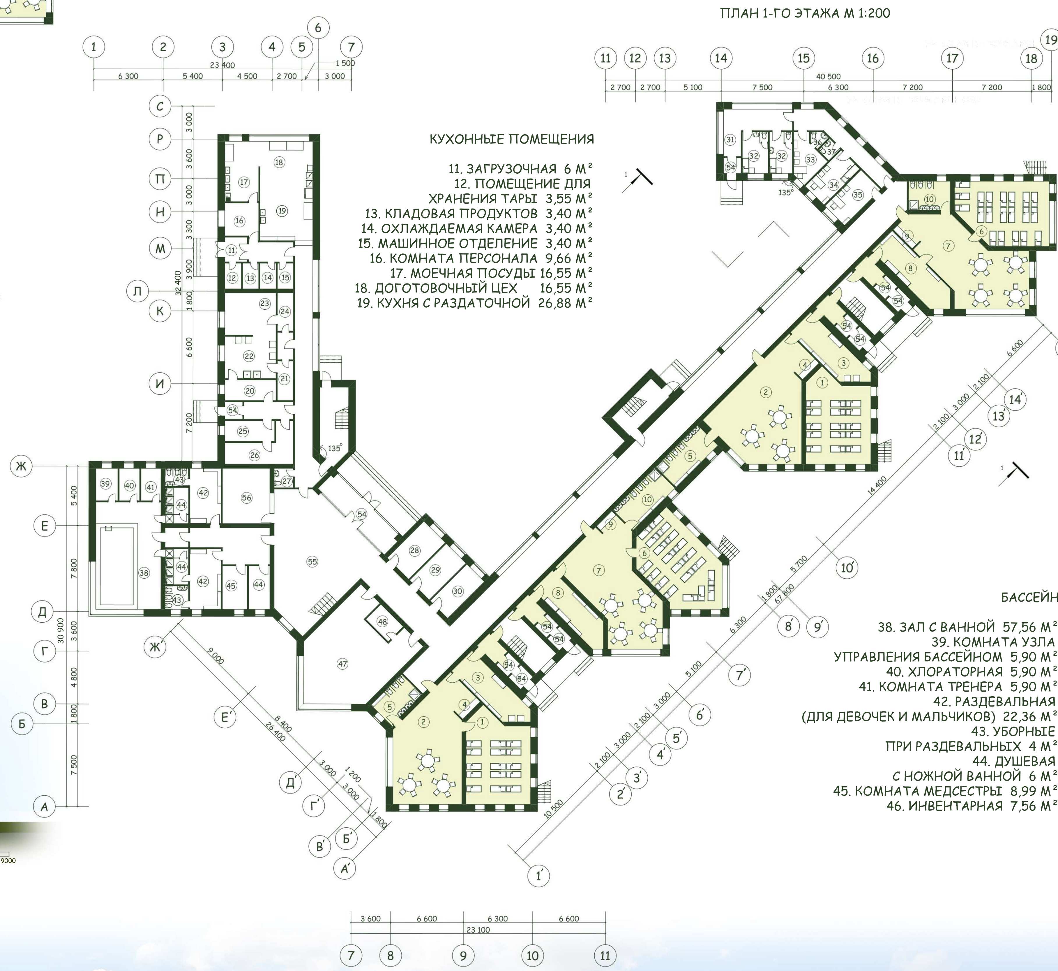
ПЛАН 1-ГО ЭТАЖА М 1:200
