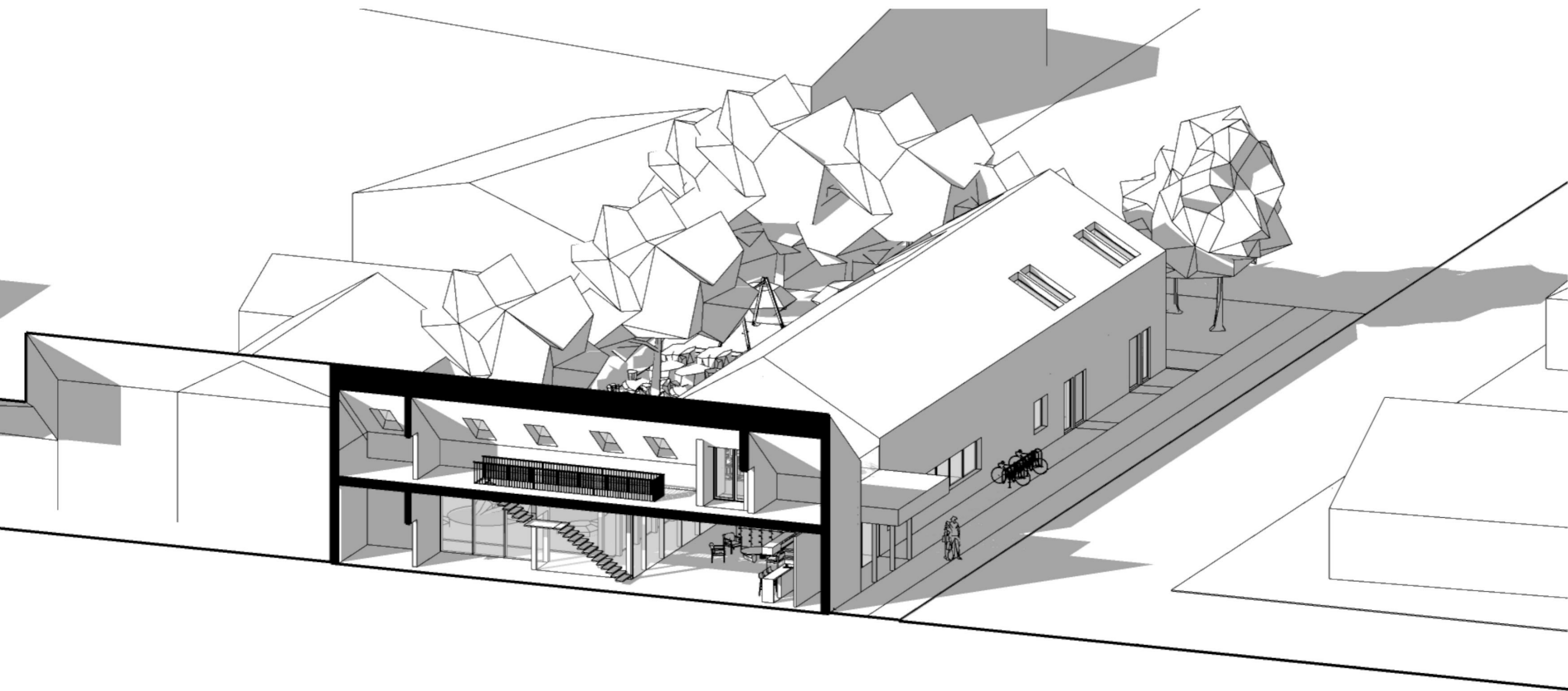
Axonometrický rez B-B
