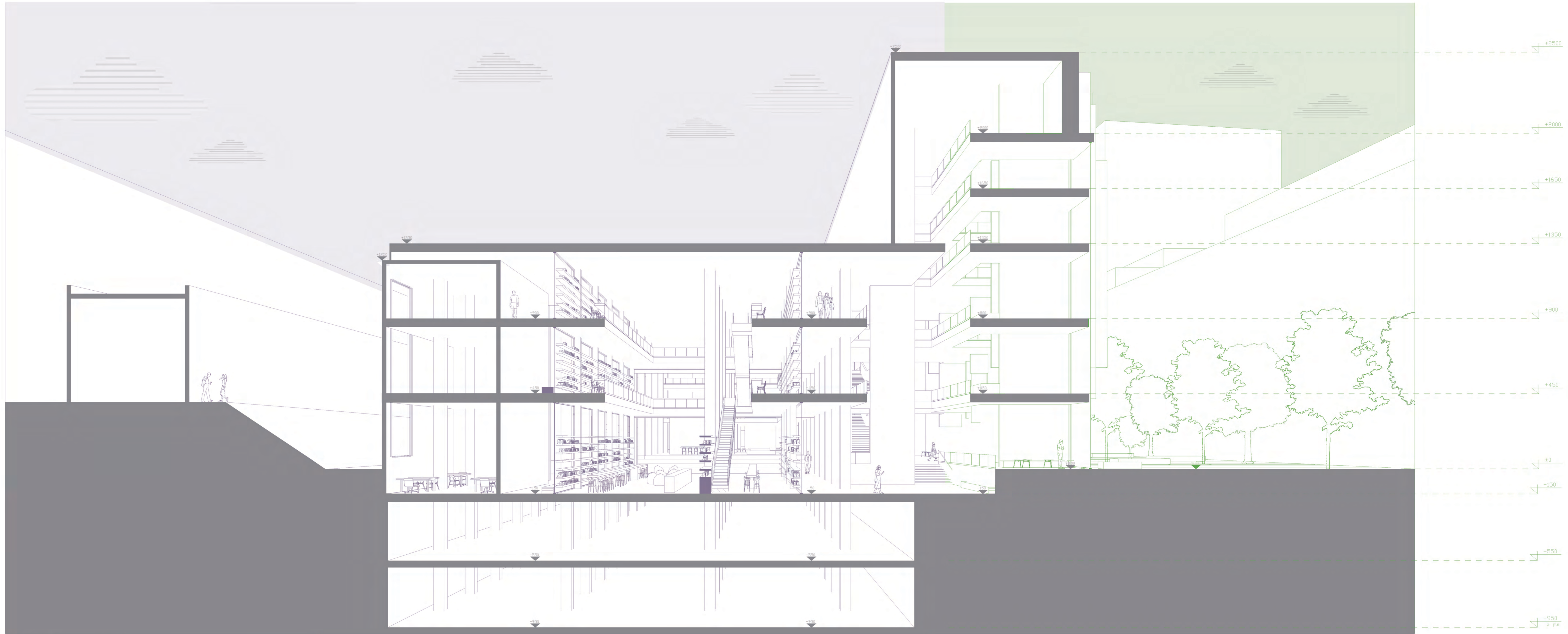
section B, 1:100
