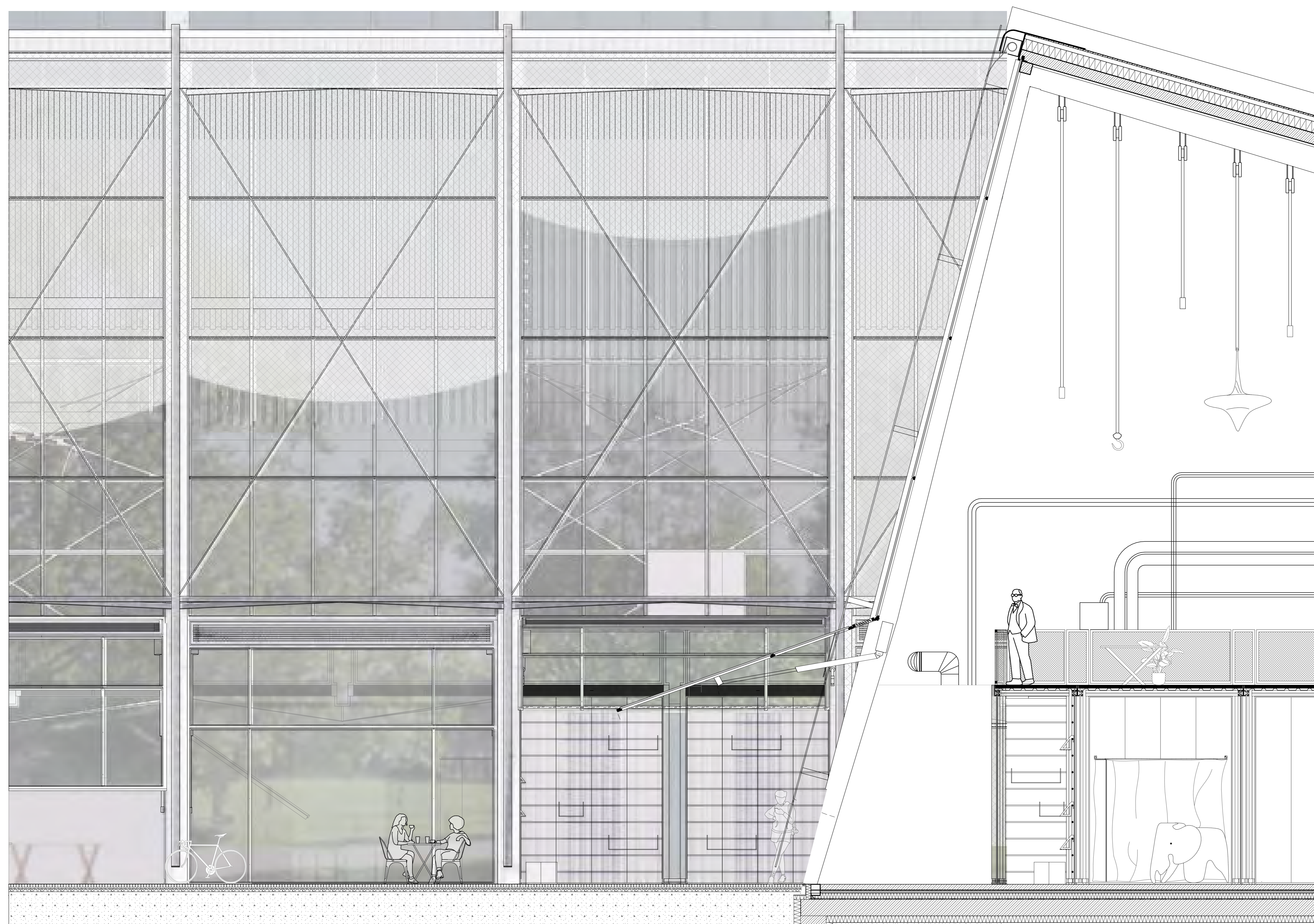
Schnittansicht 1:33
