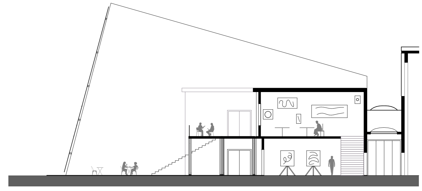
Querschnitte 1:200
