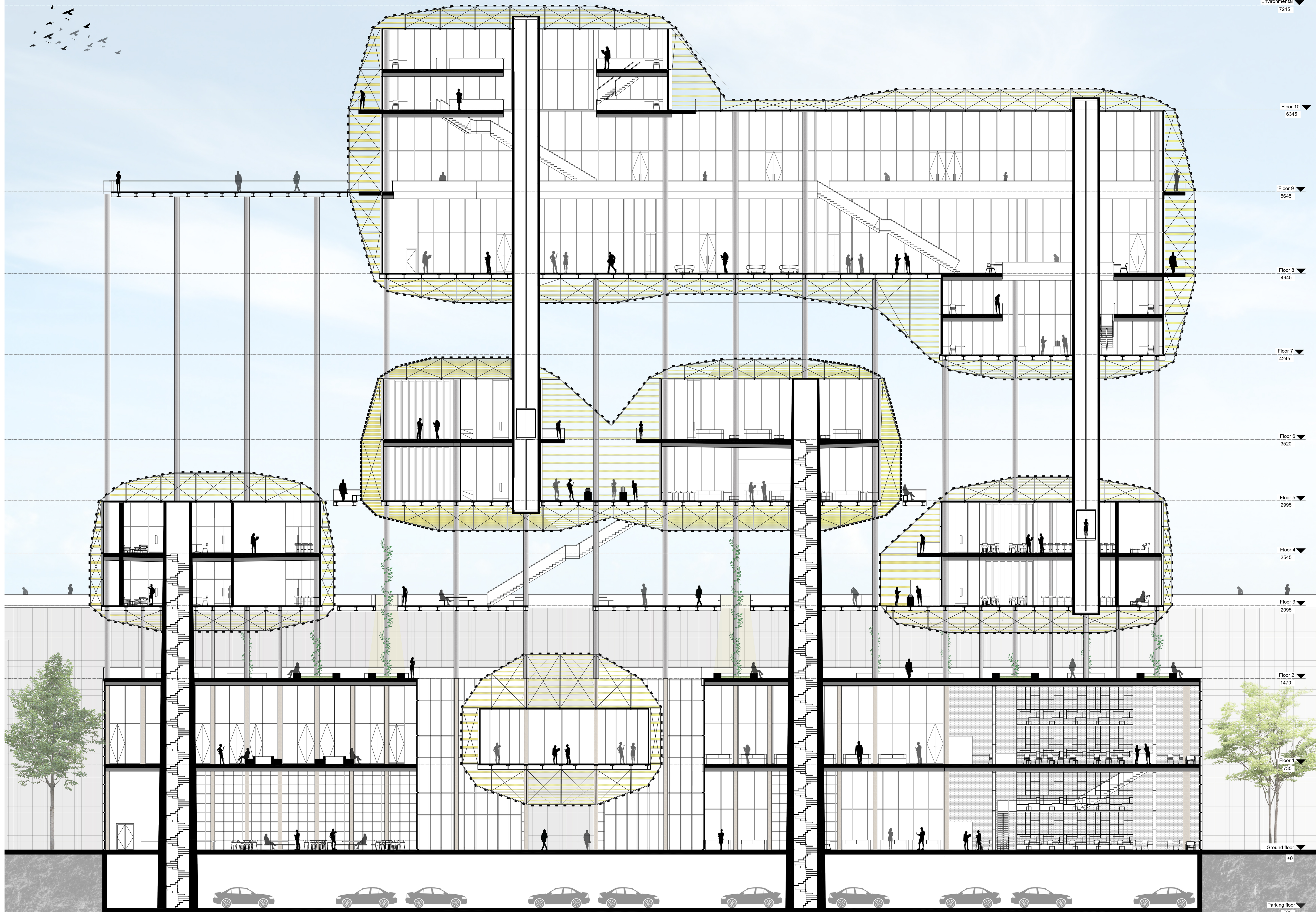
Section A-A 1:100
