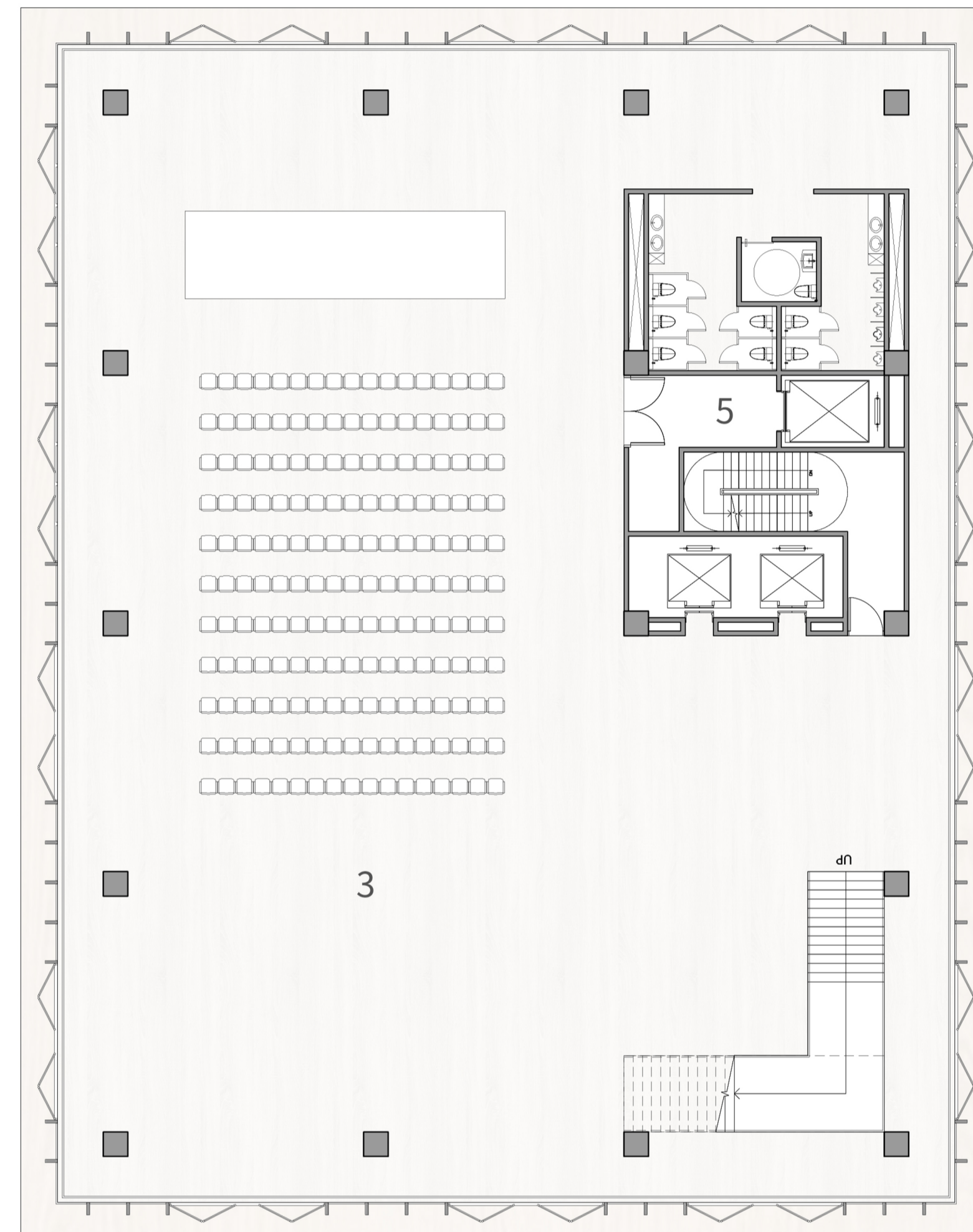
A-2F Plan Scale:1/200 ☹
