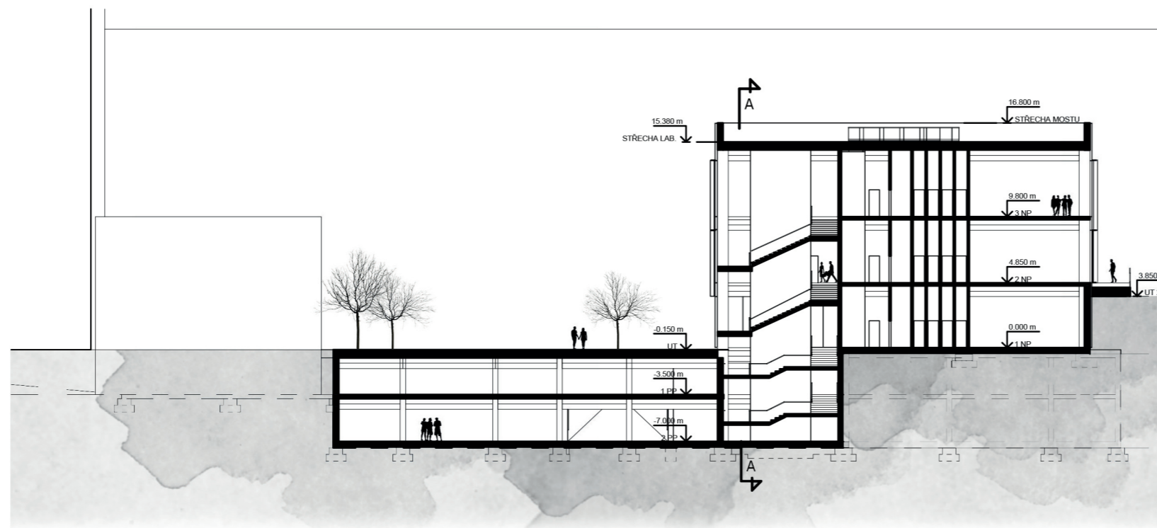
ŘEZ B-B
