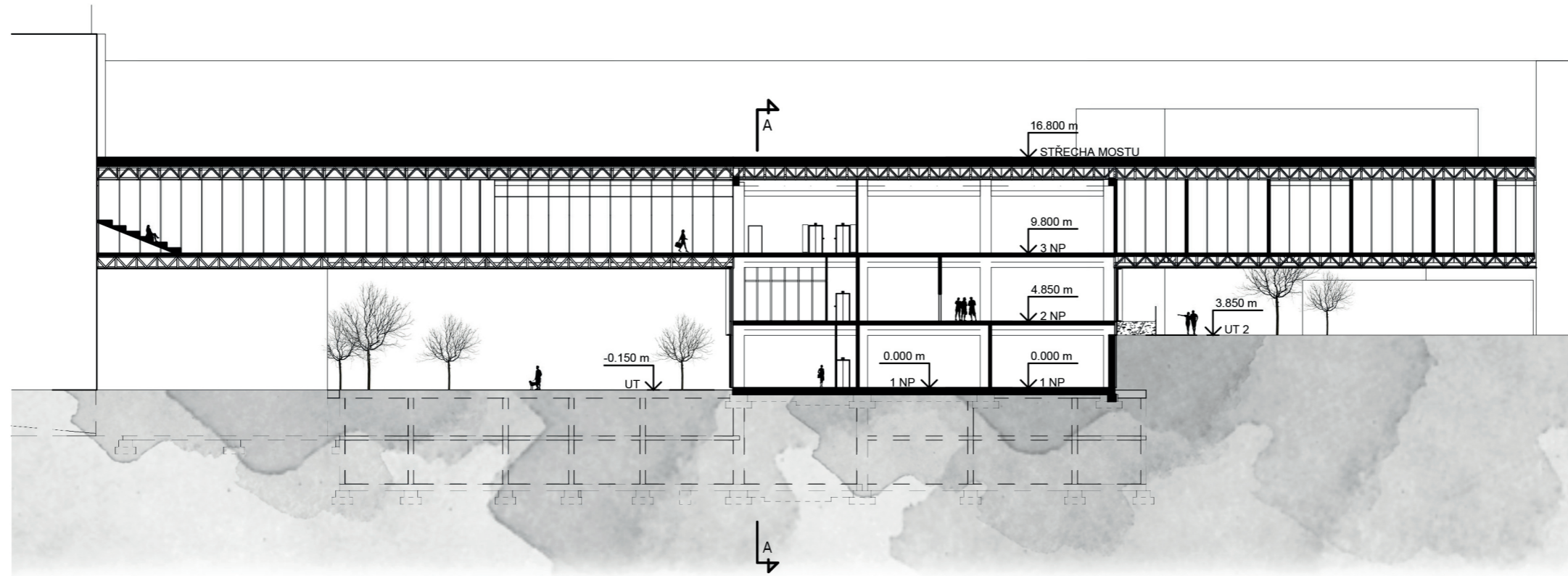
ŘEZ C-C
