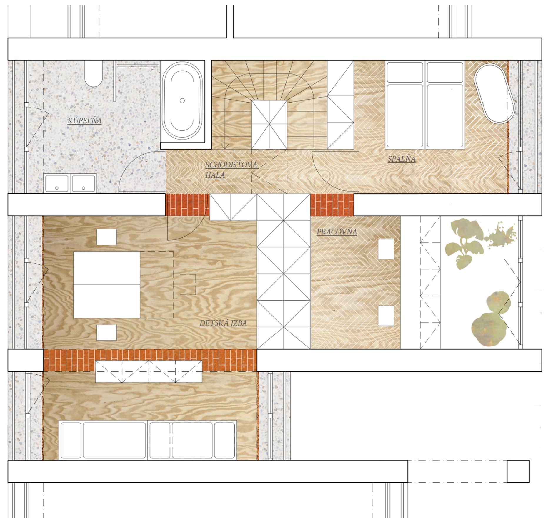
BYT B - 2. NP | 1:50
