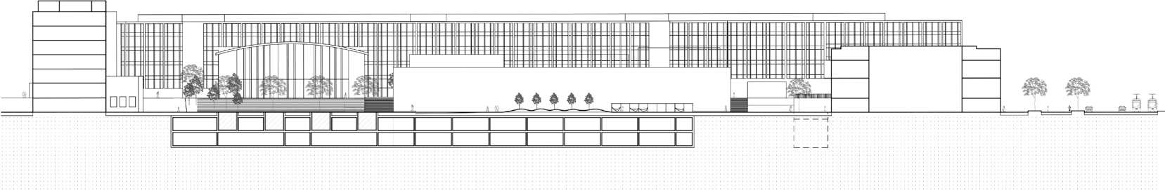
REZ B-B'
