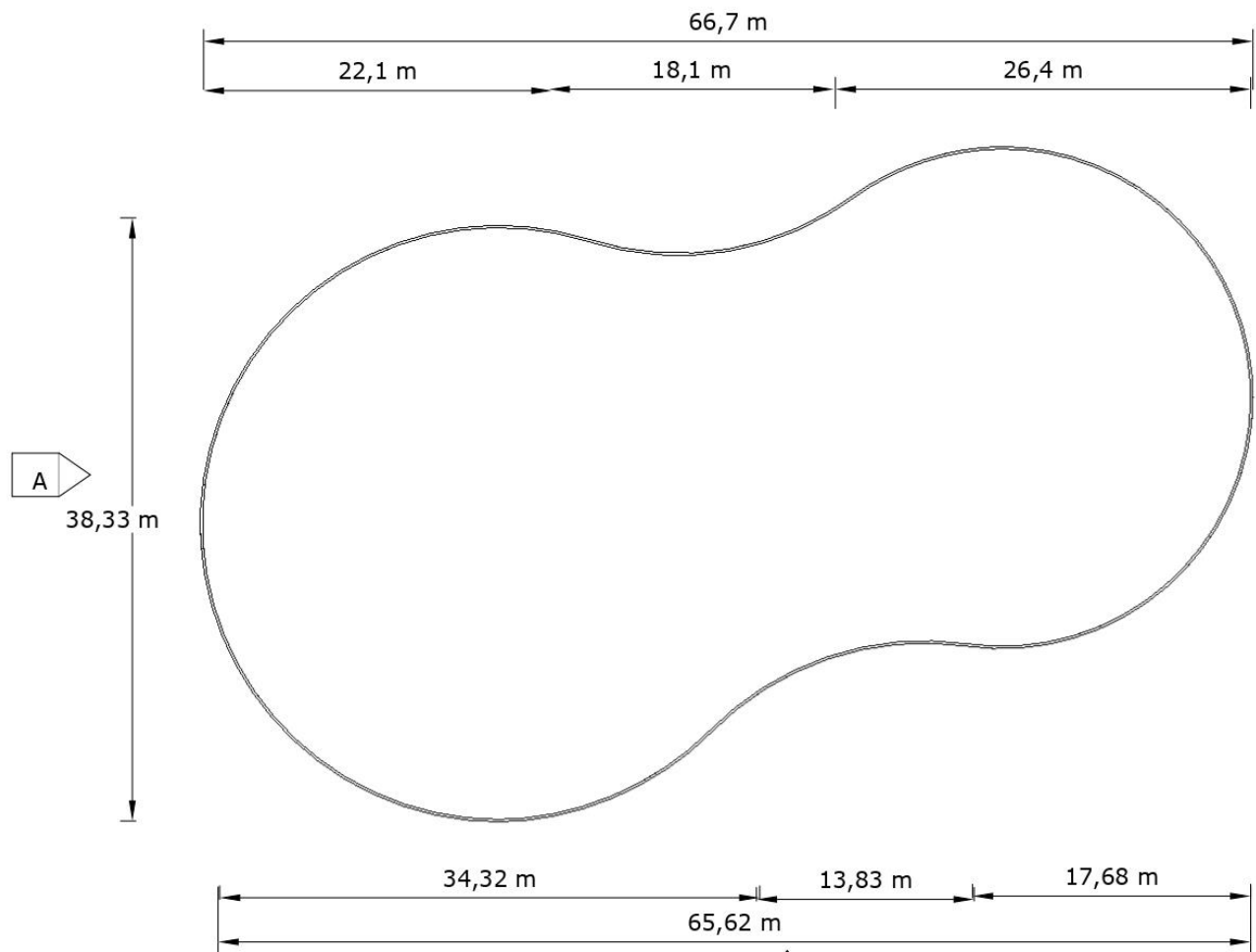
TAMPAK ATAS SECOND SKIN skala 1:400
