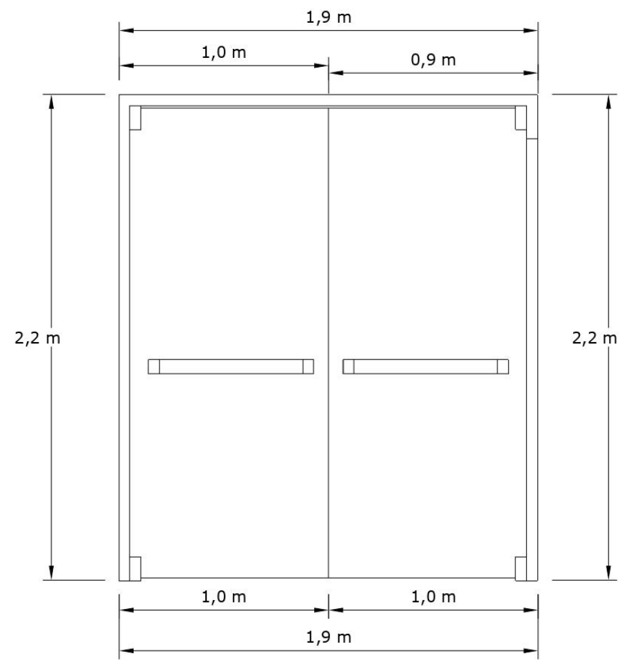
TAMPAK B PINTU 2 skala 1:20
