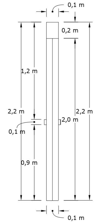
TAMPAK A PINTU 2 skala 1:20
