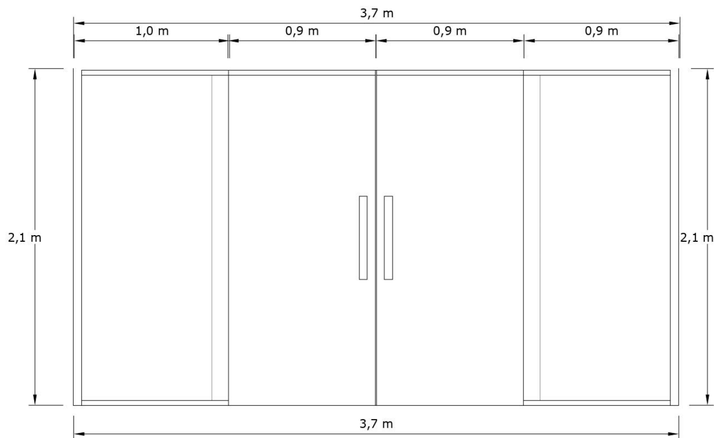
TAMPAK B PINTU 1 skala 1:20
