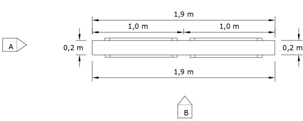
TAMPAK ATAS PINTU 2 skala 1:20
