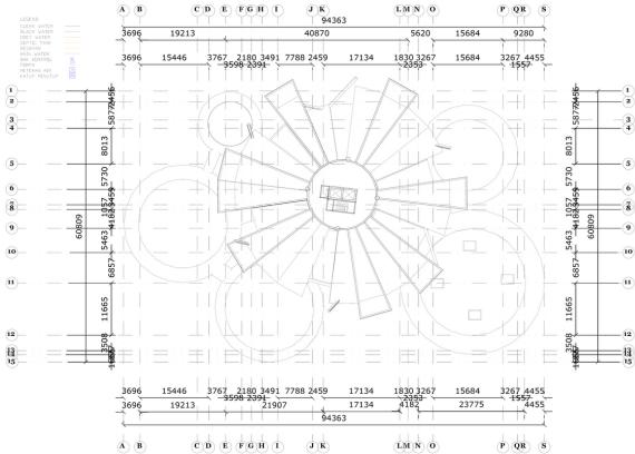
Lantai 12 SKALA 1:500
