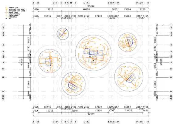
Lantai 2 SKALA 1:500
