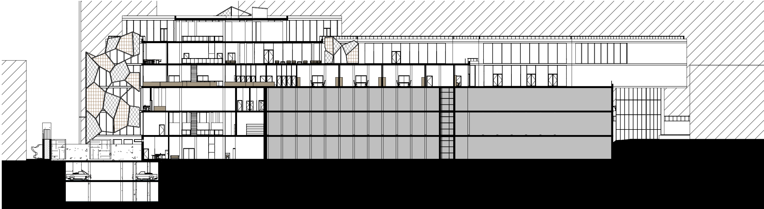
Longitude section
