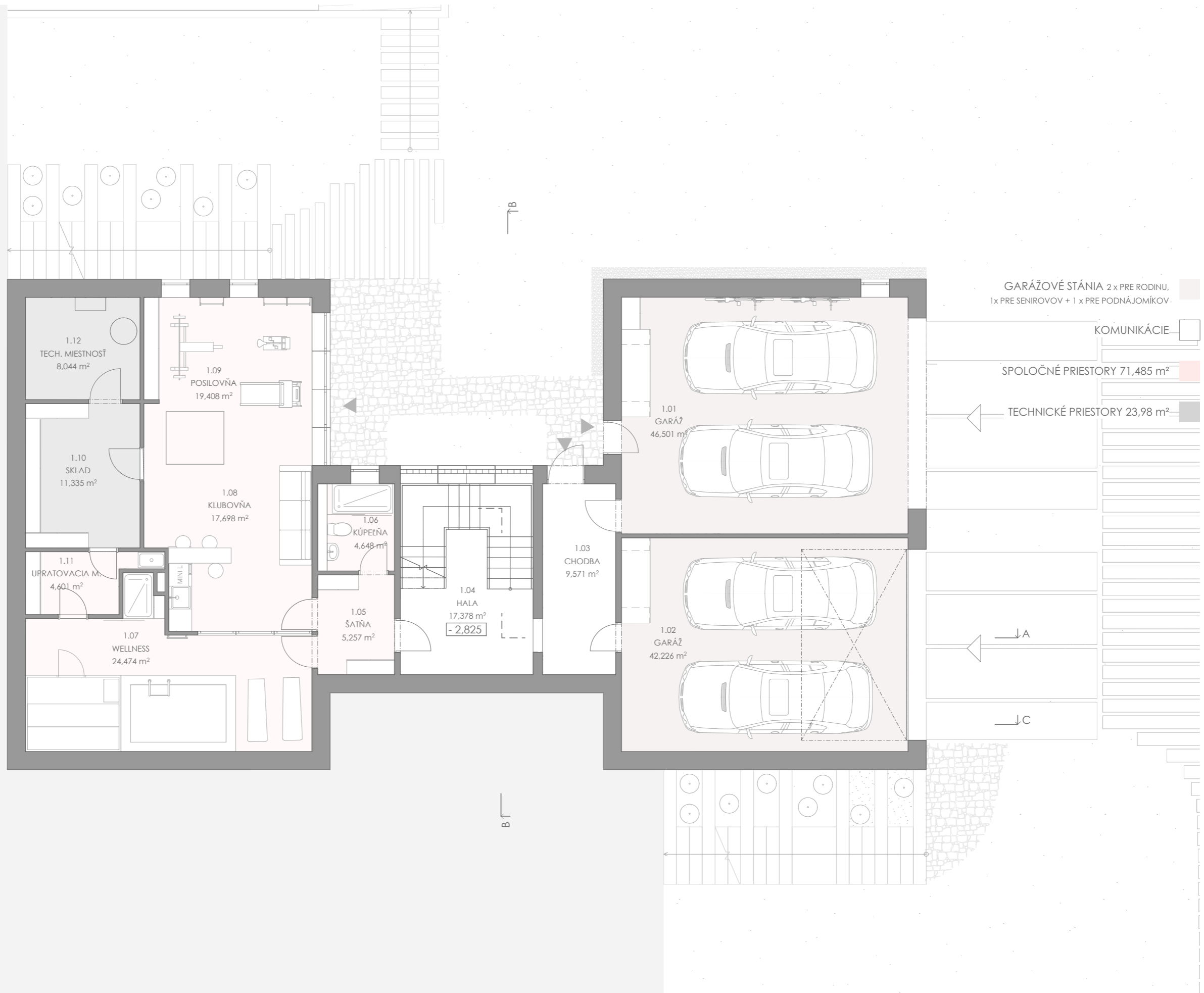
PÔDORYS 1.PP
