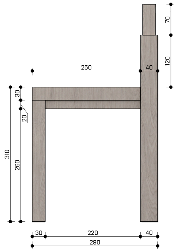
POHLED ZPRAVA
