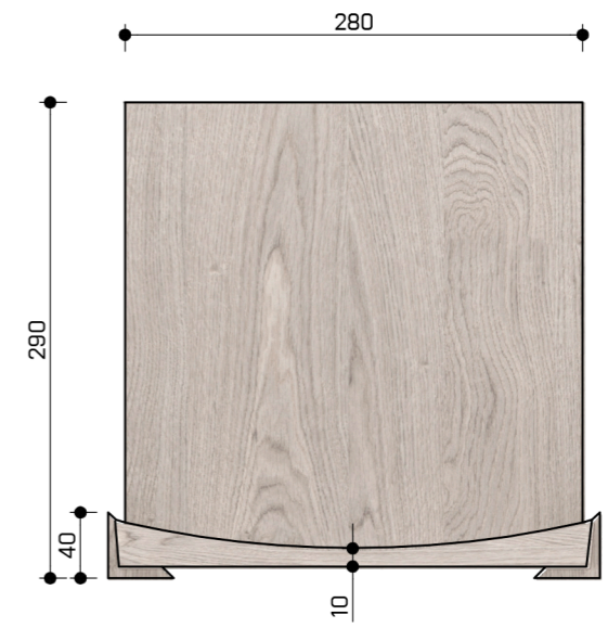
POHLED ZHORA
