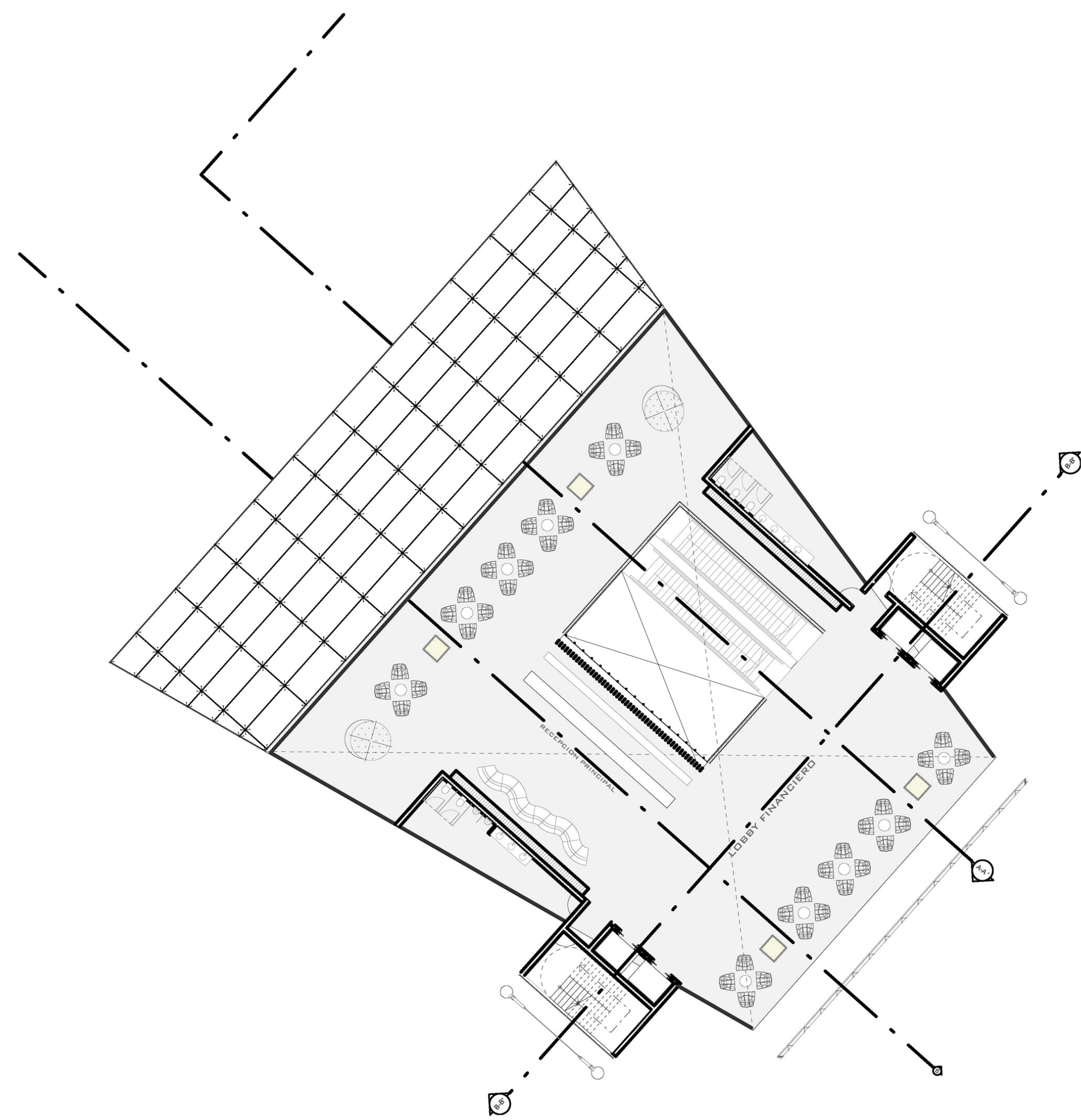
SEXTO NIVEL - LOBBY FINANCIERO ESC: 1/200
