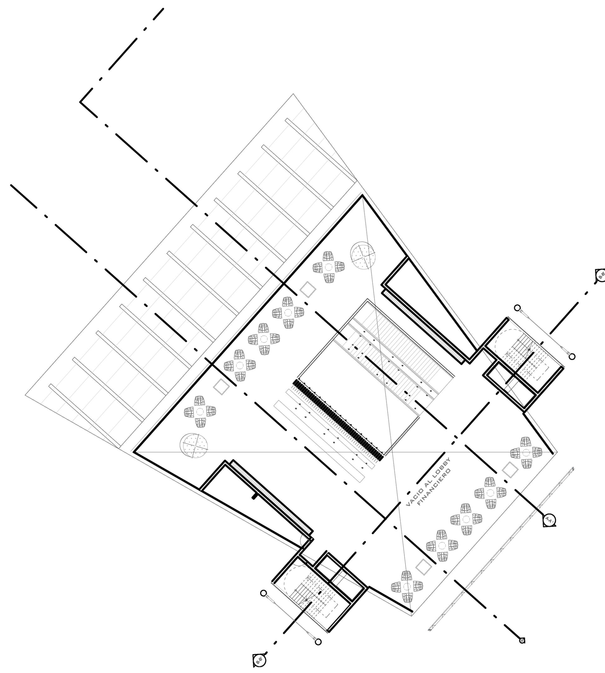
SEPTIMO NIVEL - VACIO ESC: 1/200
