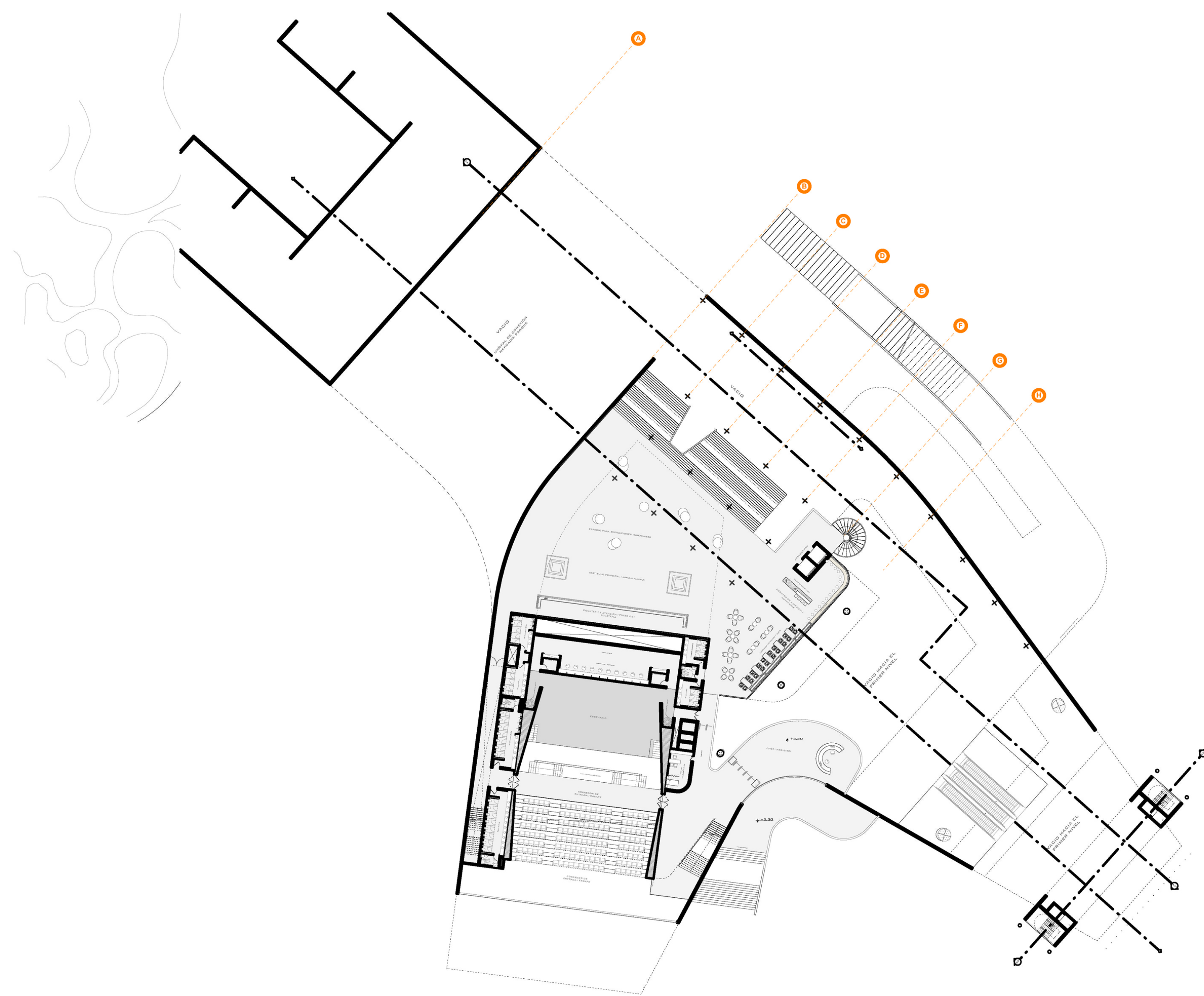
NIVEL DEL FOYER 1/500
