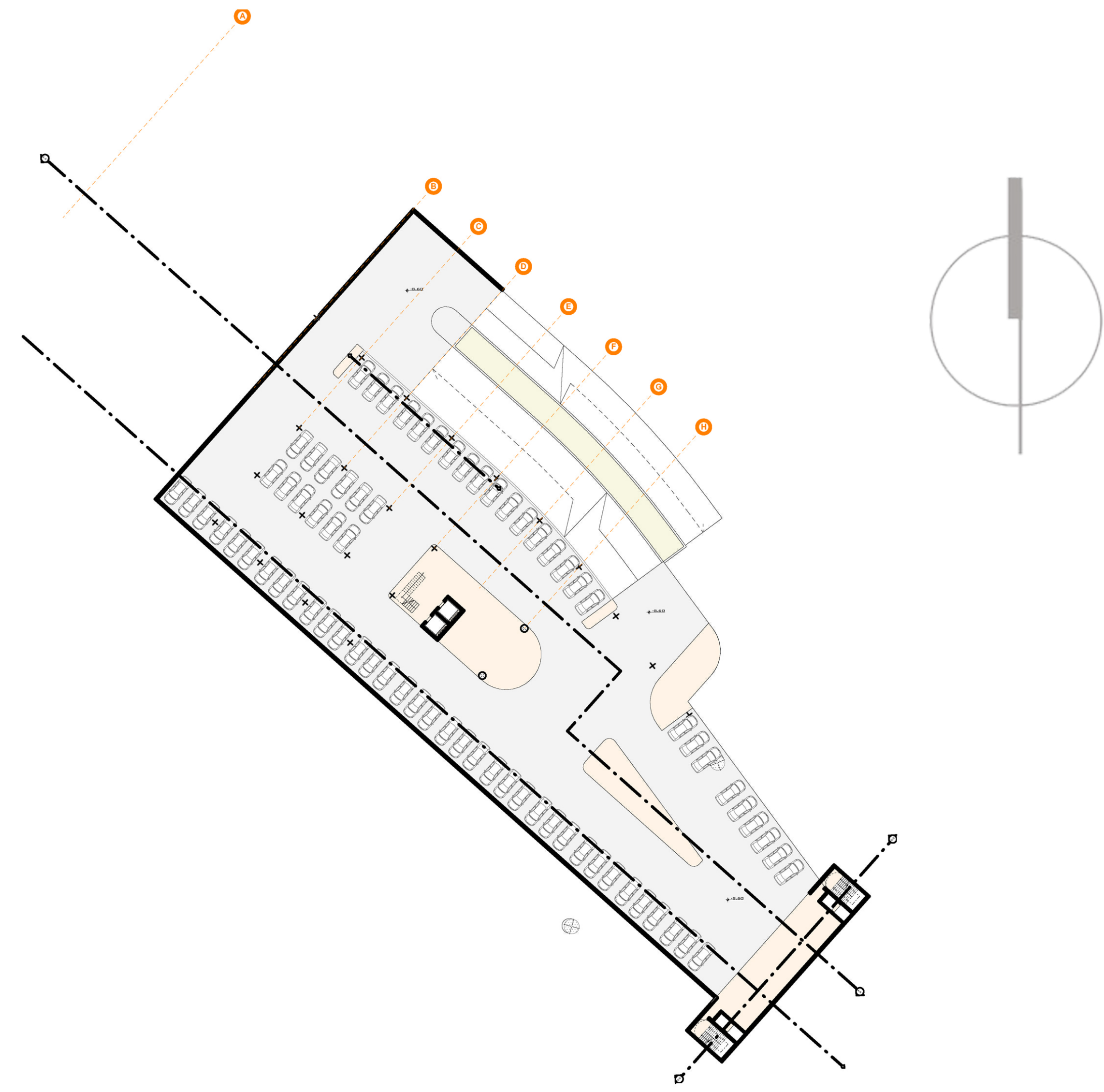
SOTANO -02 1/500
