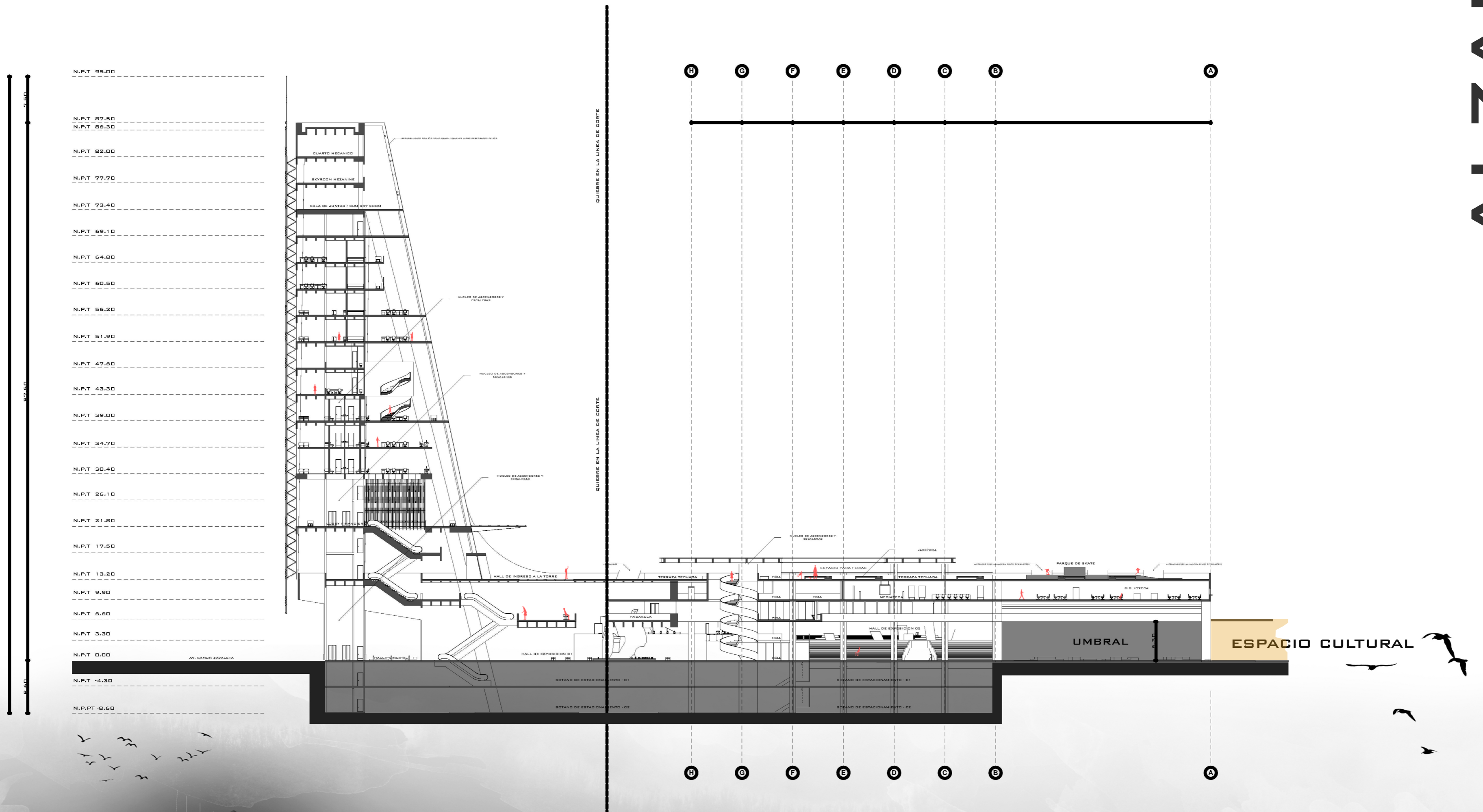
SECCION LONGITUDINAL A-A'
