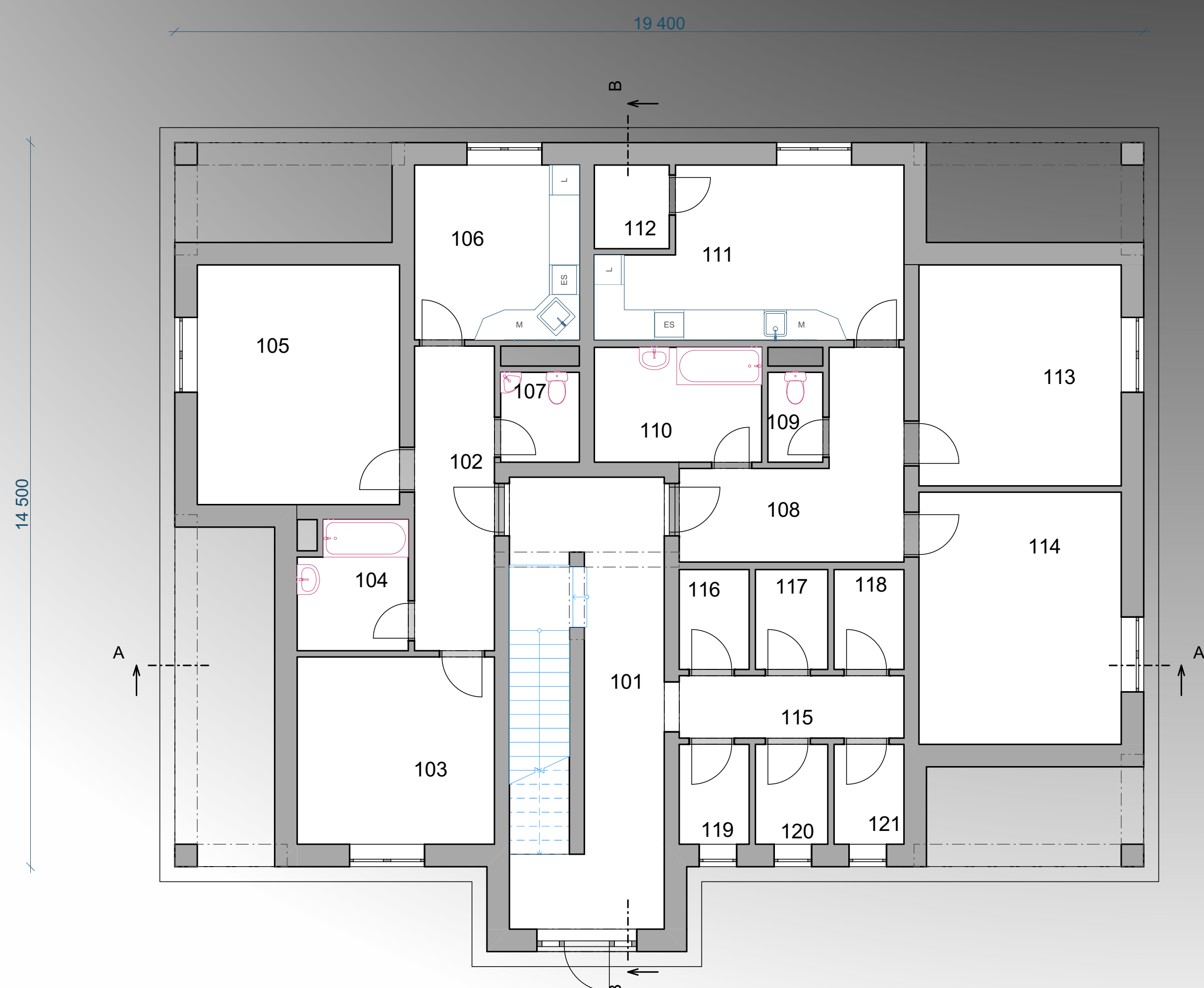
PŮDORYS
