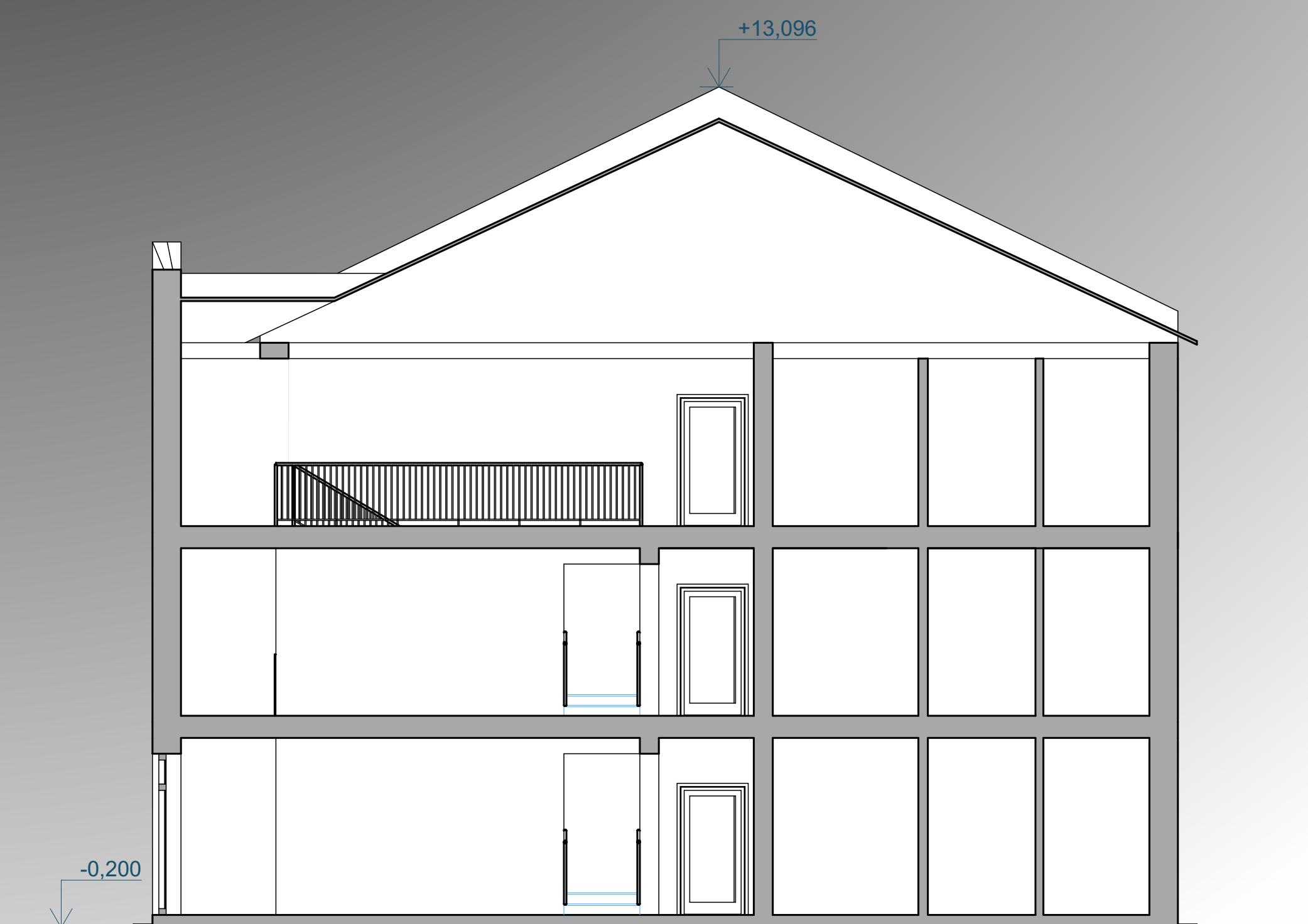
ŘEZ B-B
