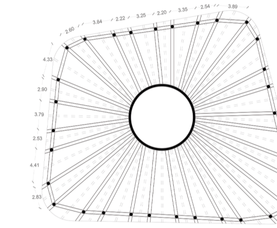
PLANTA ESTRUCTURAL
