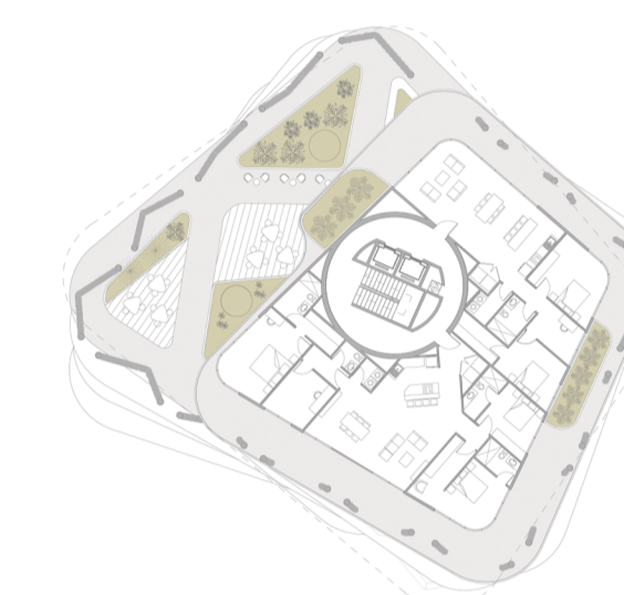
NIVEL 5
