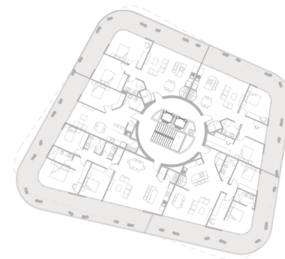
NIVEL 1
