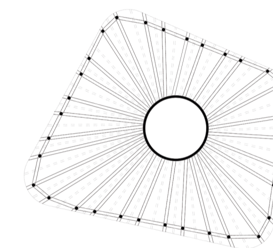
PLANTA ESTRUCTURAL
