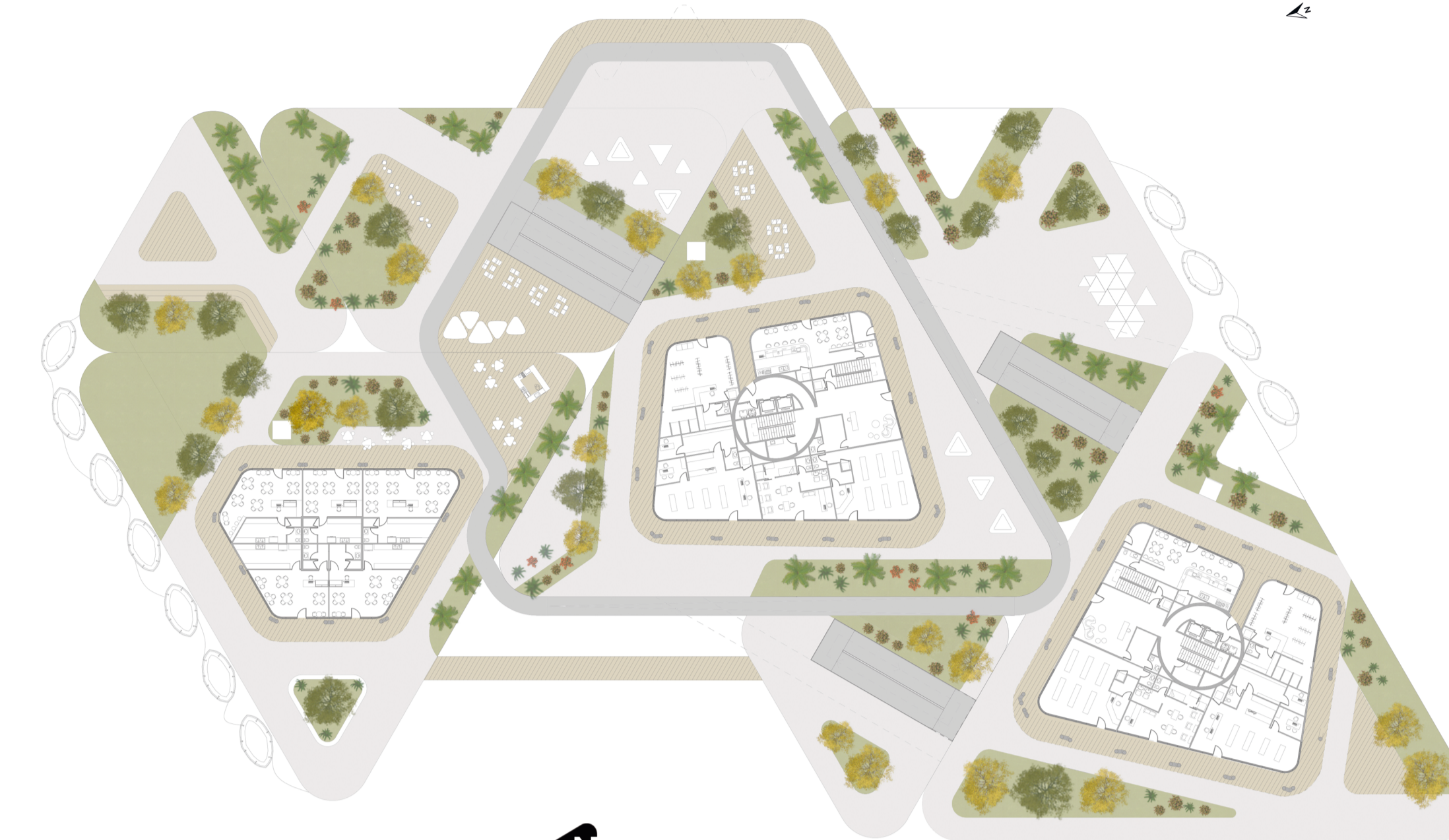
PLANTA CONJUNTO
