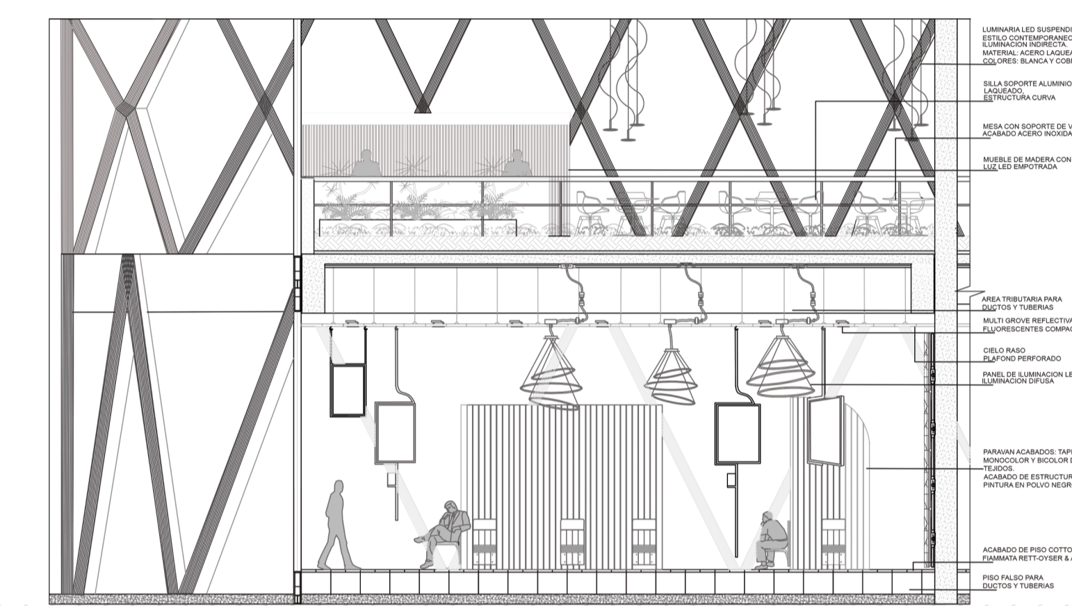
CORTE ESPACIO REPRESENTATIVO
