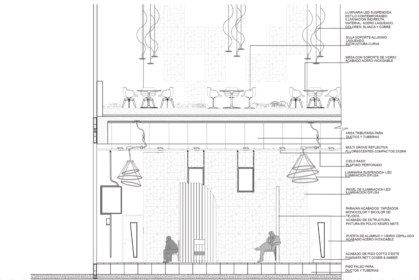
CORTE ESPACIO REPRESENTATIVO
