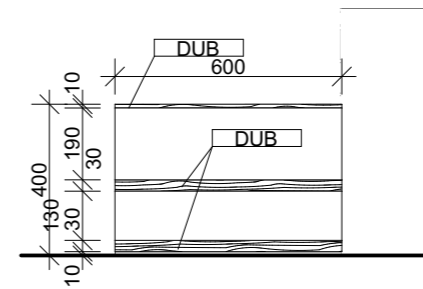
ŘEZ B3-B3'
