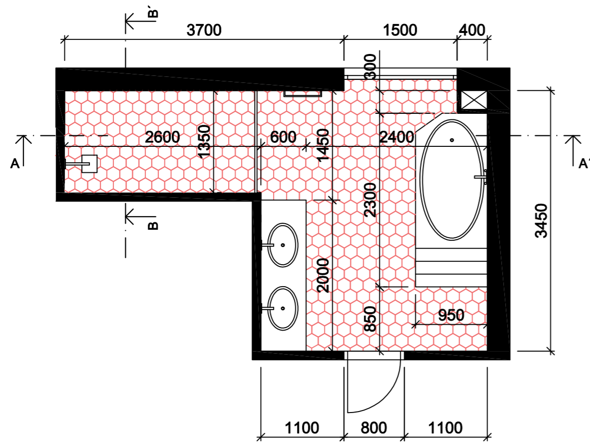
PŮDORYS
