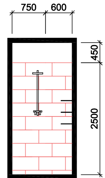
ŘEZ B-B'
