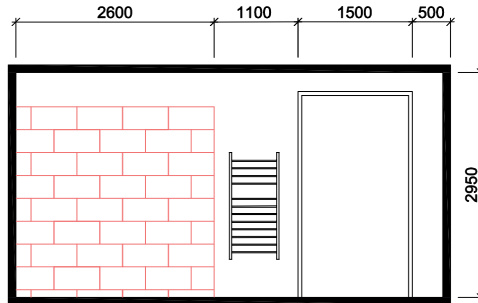
ŘEZ A-A'
