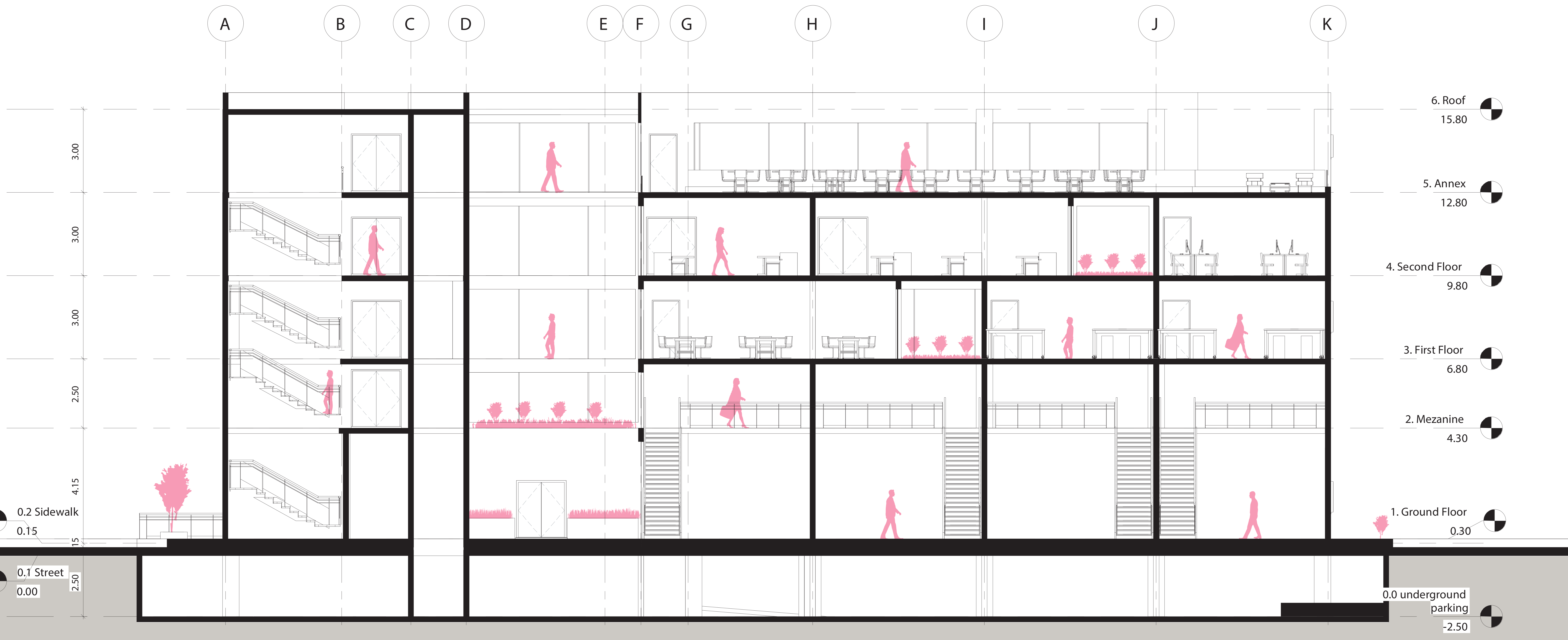
Section A-A
