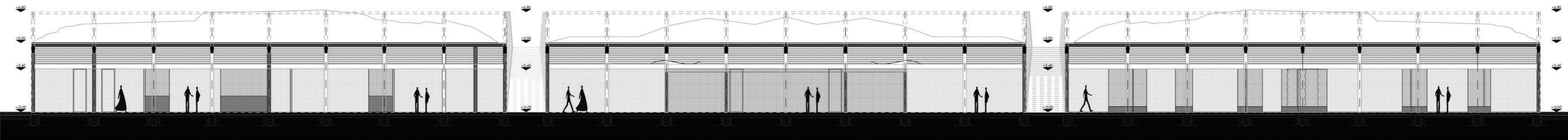
SHOW + LABO - SECTION A-A SCALE: 1/200
