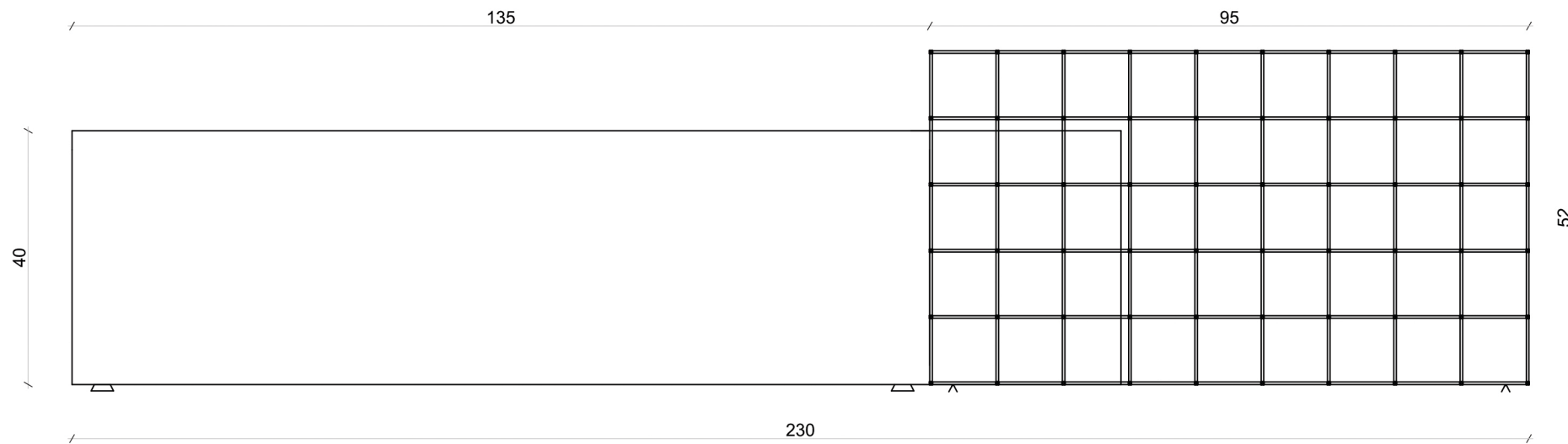
Vedere posteriora sc. 1:10
