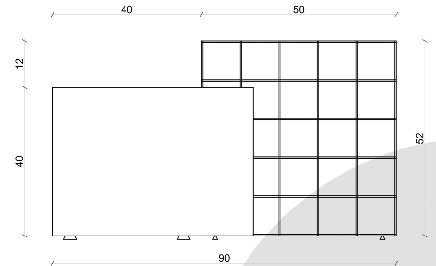
Vedere lateral dreapta sc. 1:10
