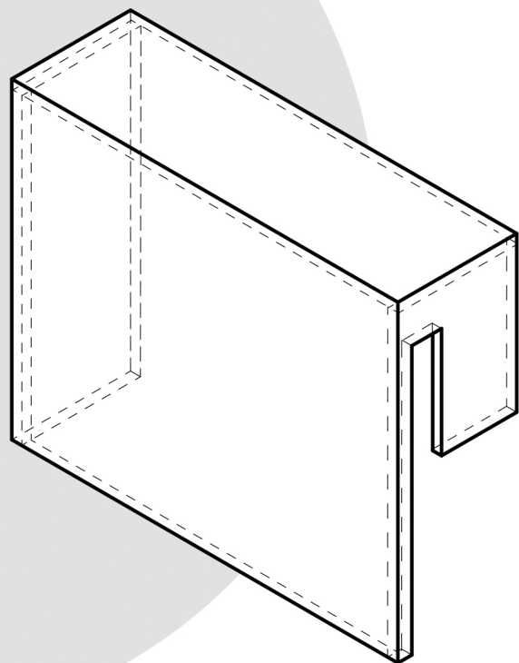
Axonometrie sc. 1:20
