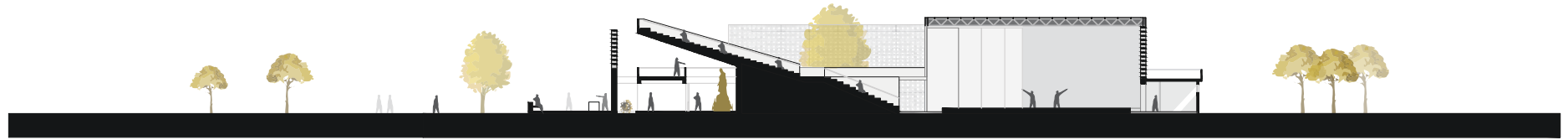
CORTE A-A
